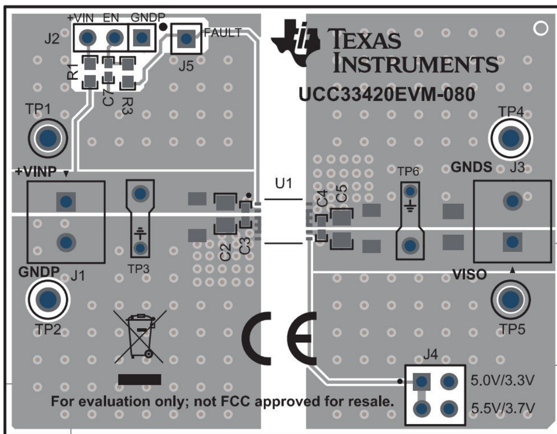
図 8-2. Layout Example
