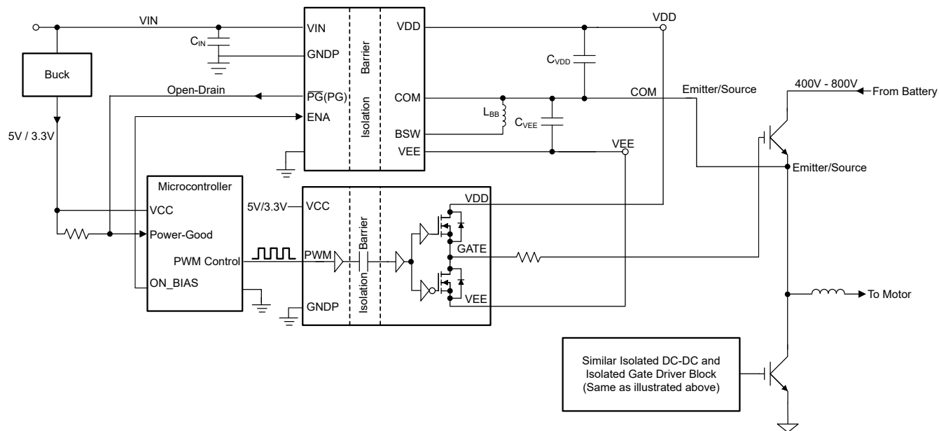
図 8-3. デュアル出力システム構成
