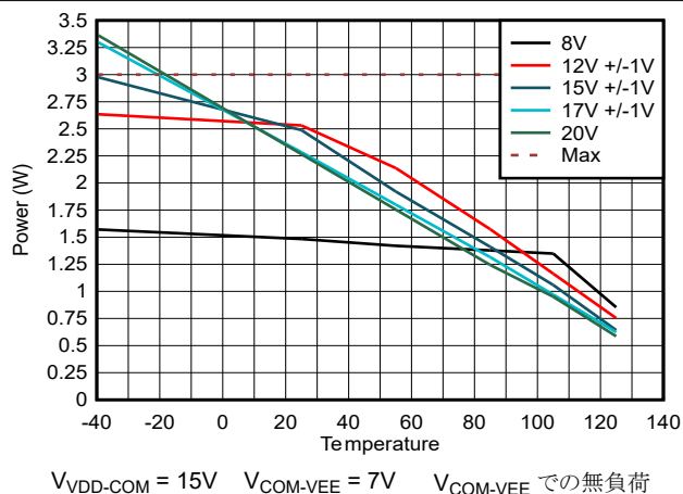
図 6-6. プリレギュレートされた入力電圧に対する SOA ディレーティング曲線
