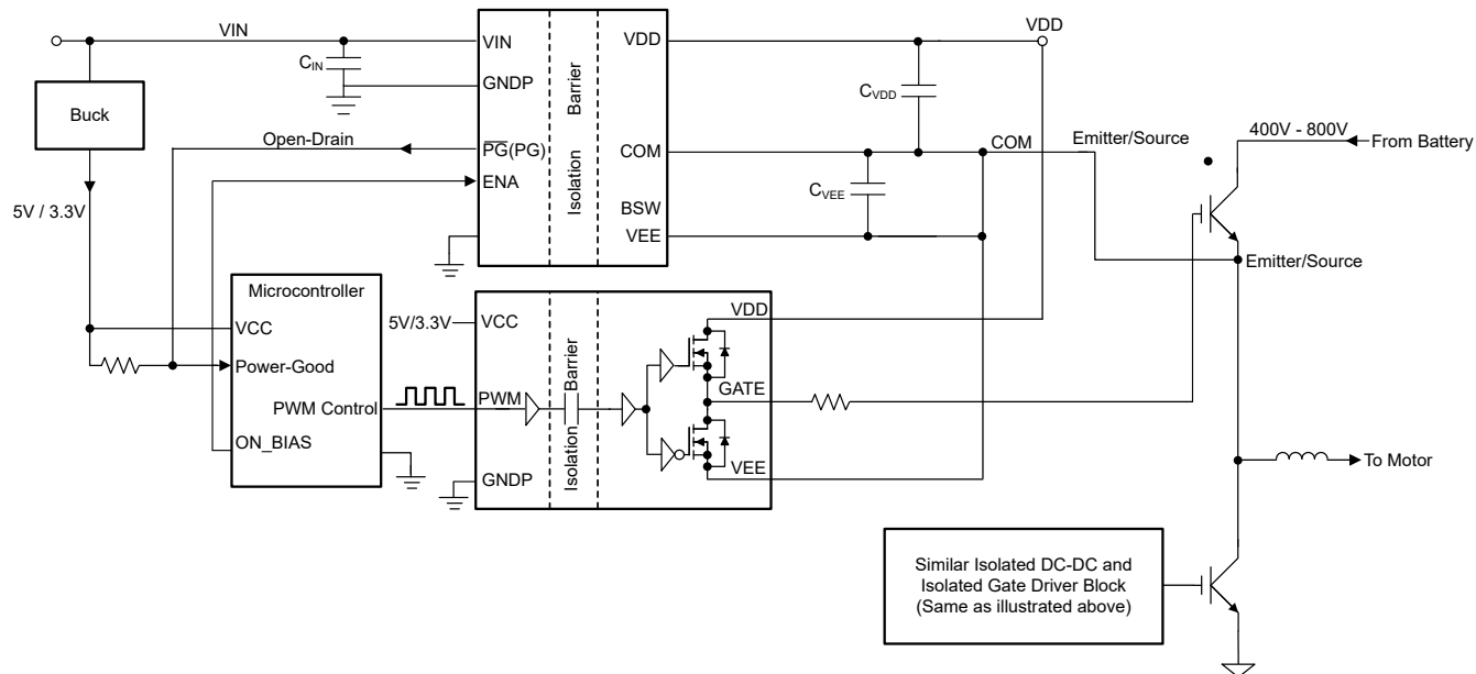
図 8-4. シングル出力システム構成
