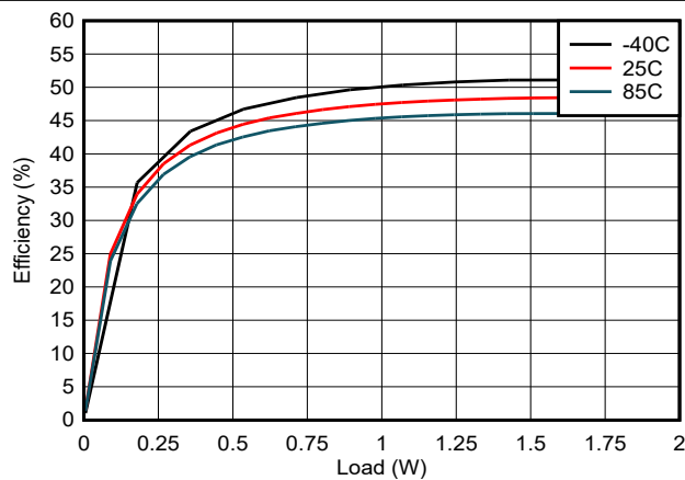
図 6-1. V_{VDD-COM} における効率と負荷との関係
