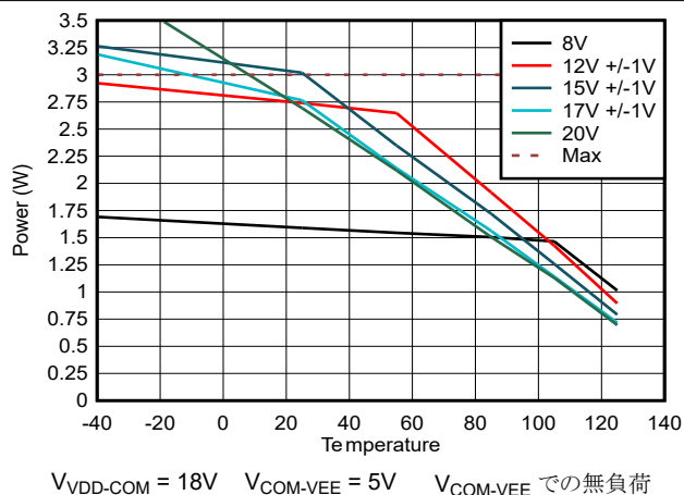
図 6-5. プリレギュレートされた入力電圧に対する SOA ディレーティング曲線
