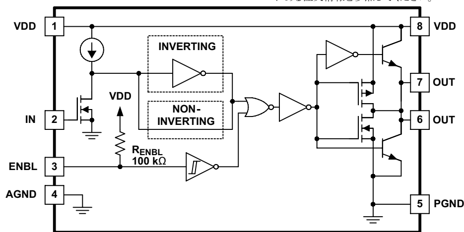
ブロック図
