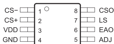
図 4-1. D or DGK Package 8-Pin SOIC or VSSOP Top View
