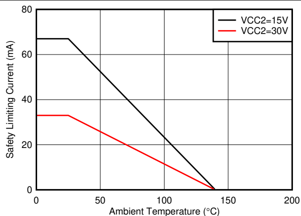
図 5-1. DWV パッケージの VDE に従う制限電流の熱特性低下曲線
