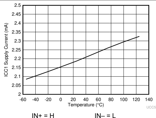
図 5-9. I_{CC1} 電源電流と温度との関係
