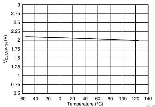
図 5-22. V_{CLAMP-TH} と温度との関係
