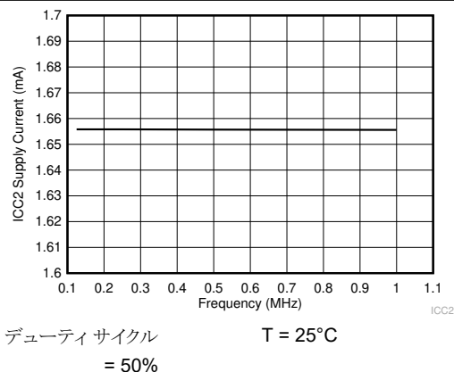
図 5-13. I_{CC2} 電源電流と入力周波数との関係
