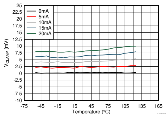
図 5-21. V_{CLAMP} と温度との関係
