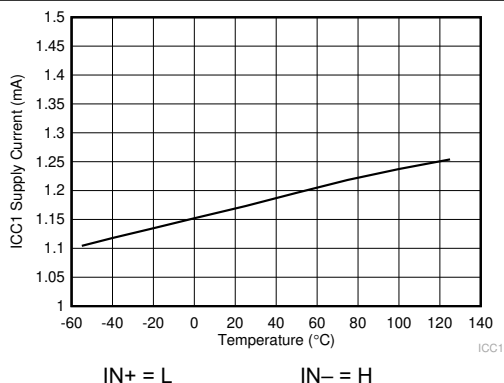
図 5-8. I_{CC1} 電源電流と温度との関係
