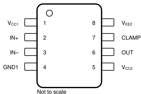
図 4-1. UCC5350MC-Q18 ピン SOIC 上面図
