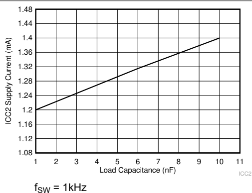
図 5-14. I_{CC2} 電源電流と負荷容量との関係
