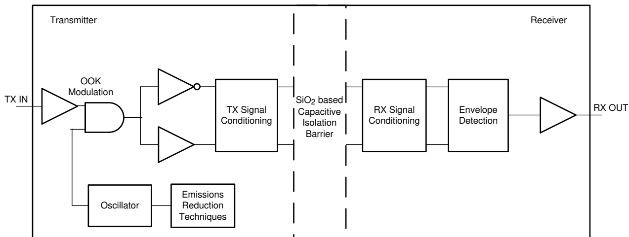
図 7-1. 容量性データチャネルの概念ブロック図
