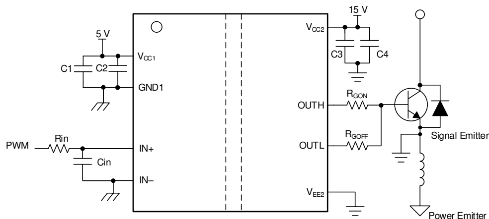
図 8-1. IGBT を駆動するための UCC5350SB-Q1 の代表的なアプリケーション回路
