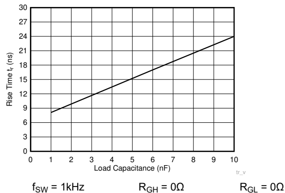
図 5-19. 立ち上がり時間と負荷容量との関係
