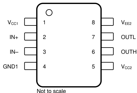
図 4-2. UCC5350SB-Q1 8 ピン SOIC 上面図
