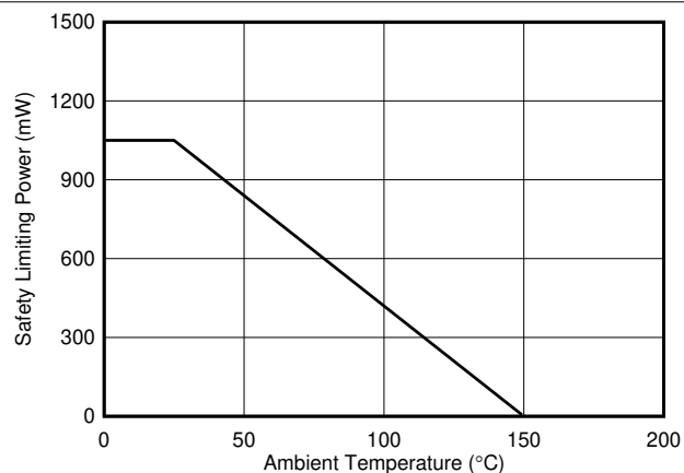
図 5-3. DWV パッケージの VDE に従う制限電力の熱特性低下曲線
