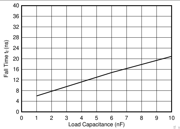
図 5-20. 立ち下がり時間と負荷容量との関係
