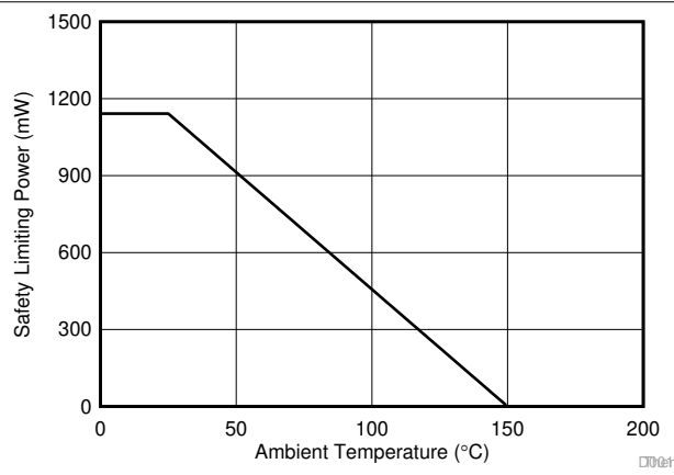
図 5-4. D パッケージの VDE に従う制限電力の熱特性低下曲線
