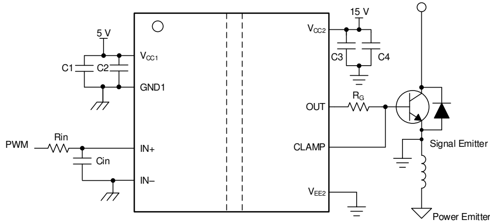
図 8-2. IGBT を駆動するための UCC5350MC-Q1 の代表的なアプリケーション回路
