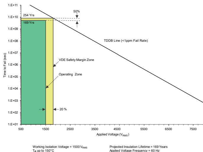
図 5-5. 絶縁寿命予測データ
