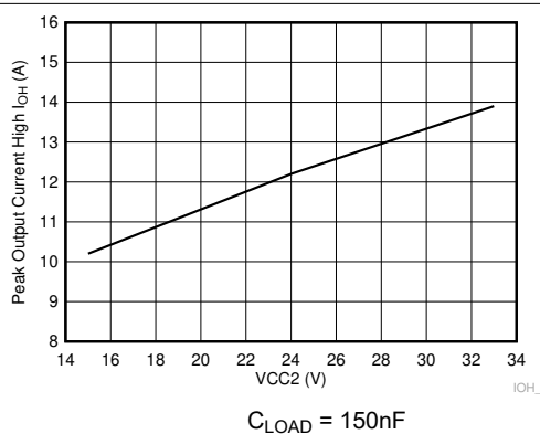
図 5-6. 出力 High の駆動電流と出力電圧との関係
