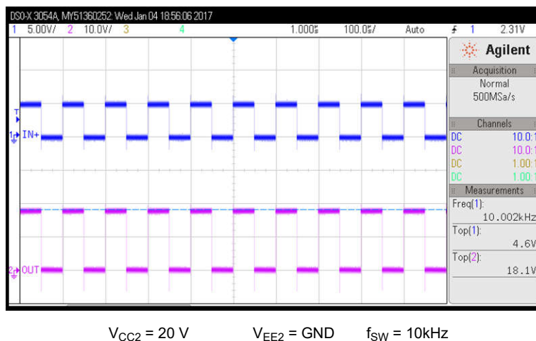
図 8-5. PWM 入力とゲート電圧波形
