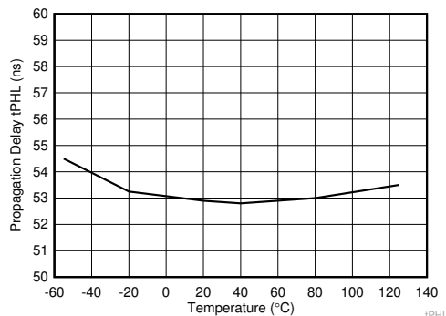
図 5-18. 伝搬遅延 t_{PHL} と温度との関係
