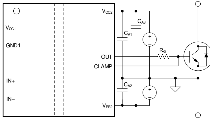
図 8-4. 2 つの絶縁型バイアス電源による負のバイアス
