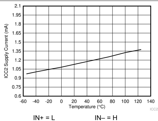
図 5-11. I_{CC2} 電源電流と温度との関係
