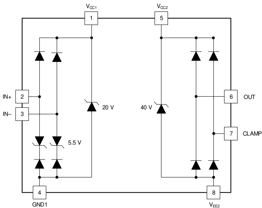
図 7-9. ESD 構造の「M」バージョン
