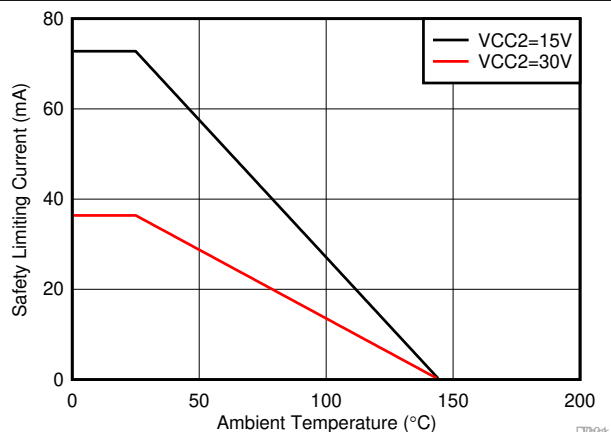
図 5-2. D パッケージの VDE に従う制限電流の熱特性低下曲線
