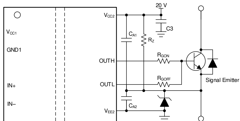
図 8-3. 絶縁型バイアス電源の出力に接続したツェナー ダイオードによる負バイアス
