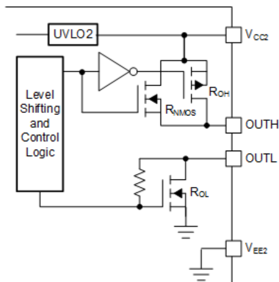
図 7-5. 出力段— S バージョン
