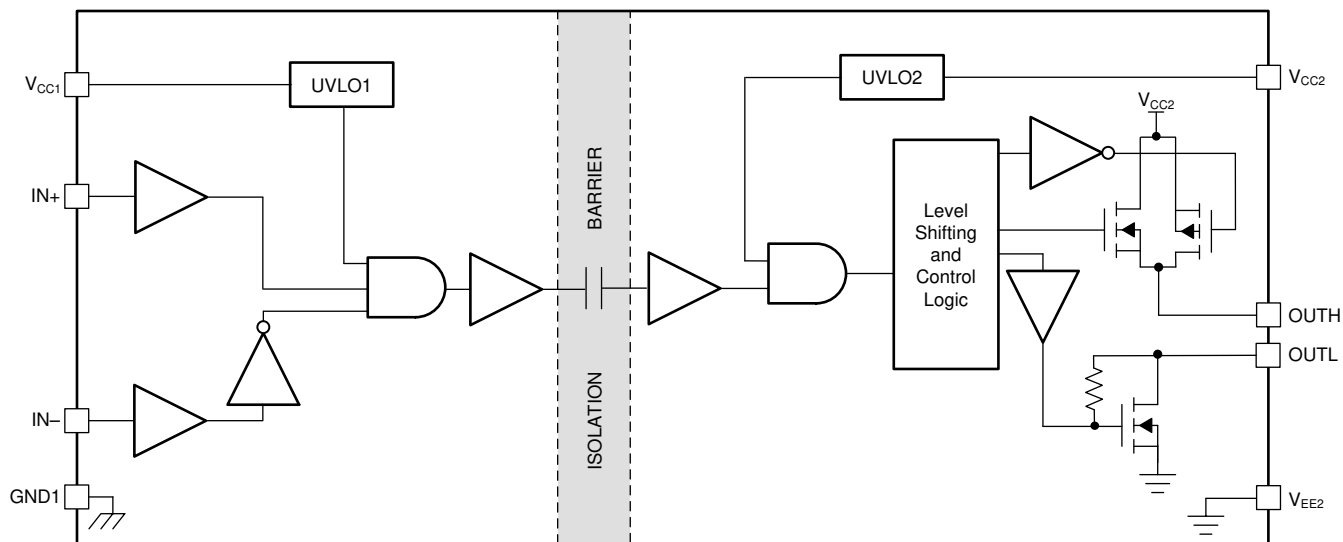
図 7-3. 機能ブロック図 — 分割出力
