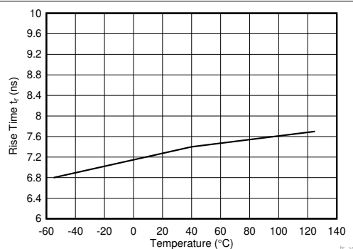
図 5-15. 立ち上がり時間と温度との関係
