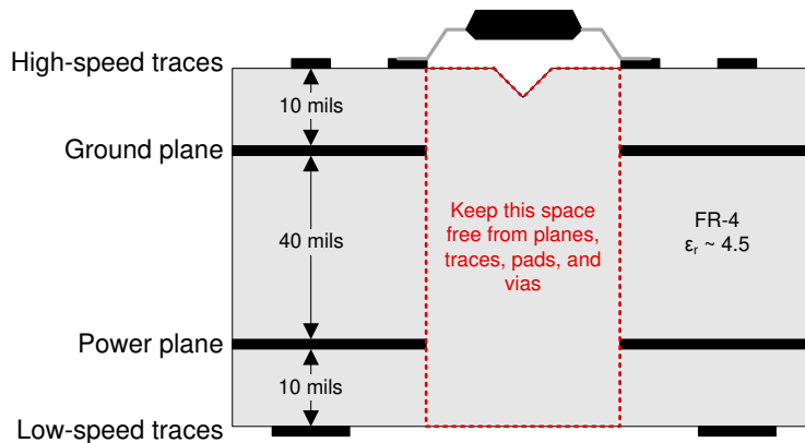
図 10-5. 推奨されるレイヤ・スタック
