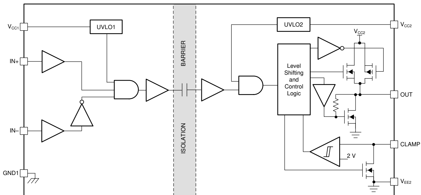
図 7-4. 機能ブロック図 — ミラークランプ
