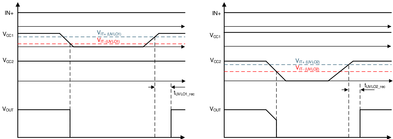
図 7-7. UVLO 機能
