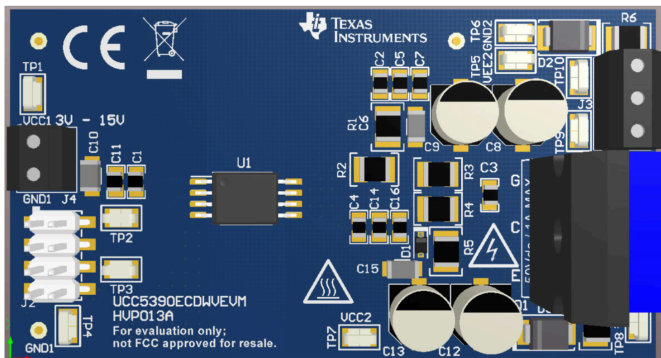
図 10-4. PCB の 3D 図
