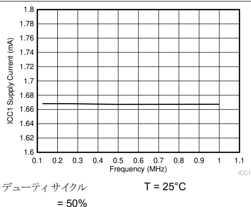
図 5-10. I_{CC1} 電源電流と入力周波数との関係
