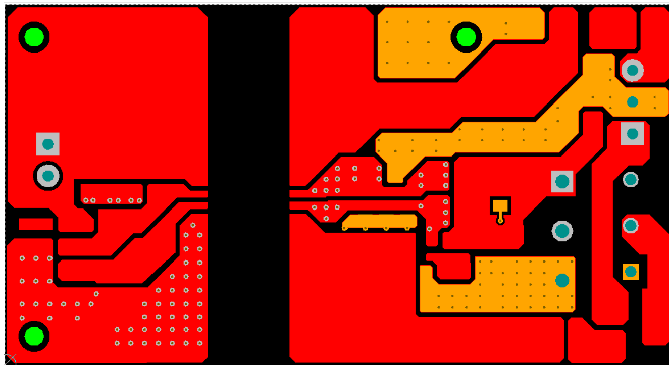
図 10-2. 上層のパターンと銅箔
