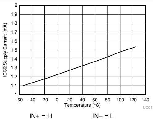
図 5-12. I_{CC2} 電源電流と温度との関係
