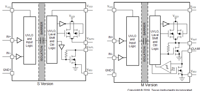
機能ブロック図 (S、M バージョン)
