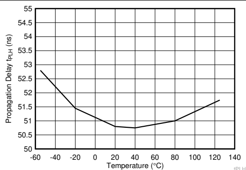
図 5-17. 伝搬遅延 t_{PLH} と温度との関係
