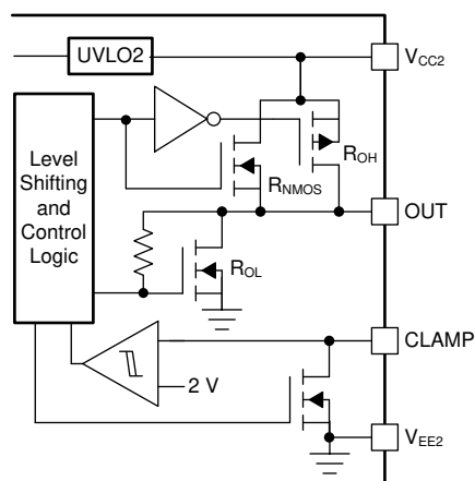
図 7-6. 出力段— M バージョン
