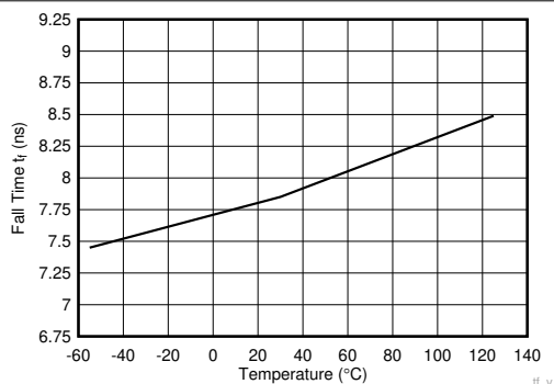
図 5-16. 立ち下がり時間と温度との関係
