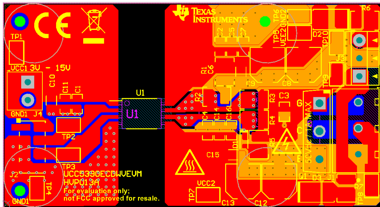
図 10-1. レイアウト例
