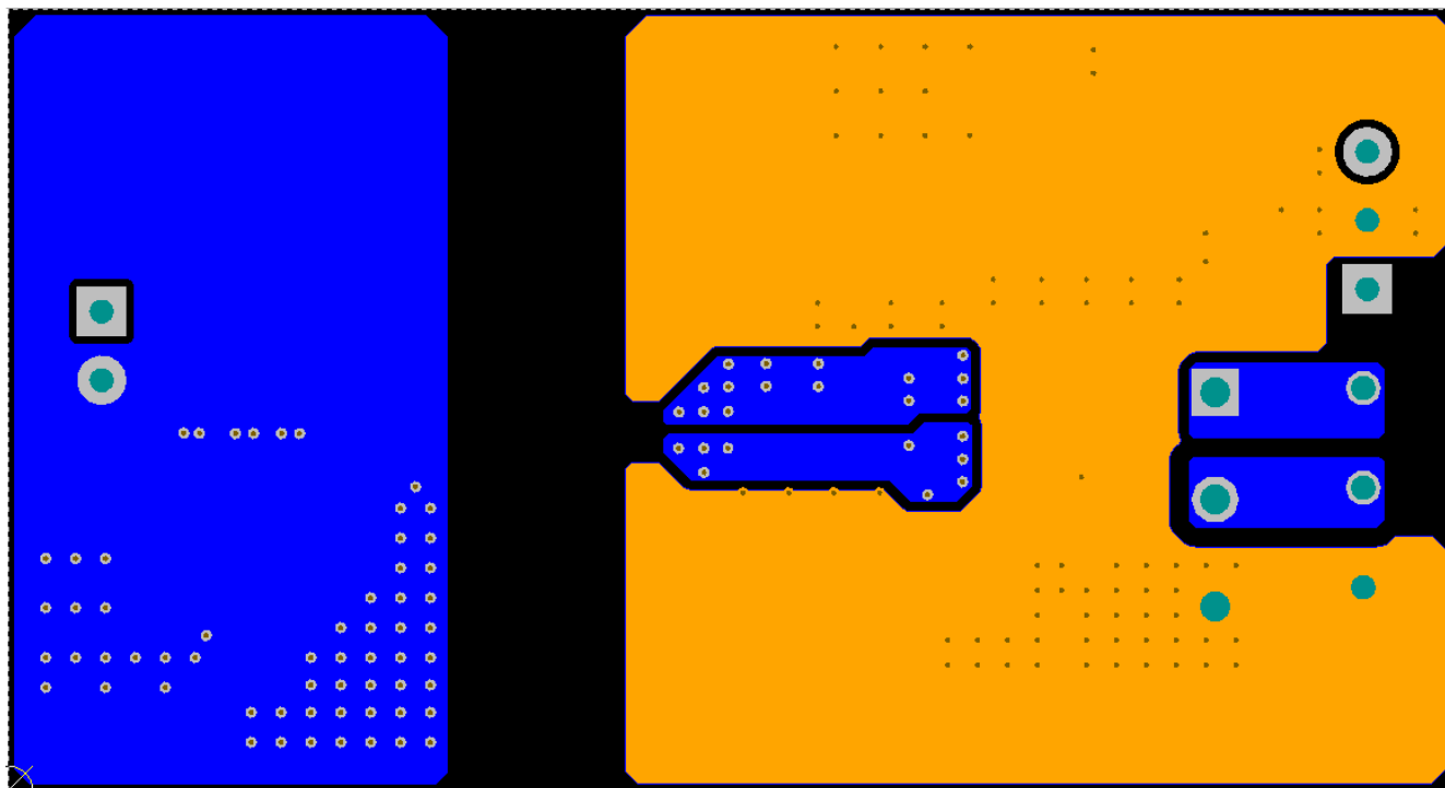
図 10-3. 下層のパターンと銅箔 (反転)
