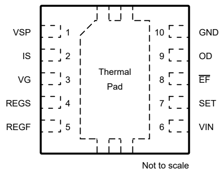
図 4-2. DRC Package, 10-Pin VSON (Top View)
