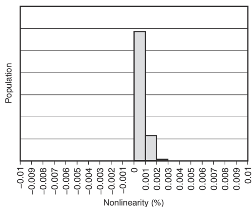
図 5-7. Nonlinearity Distribution
