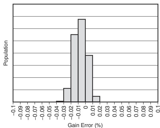
図 5-8. Gain Error Distribution
