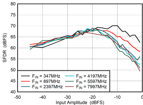
5-59. DES Mode: SFDR vs Input Amplitude
