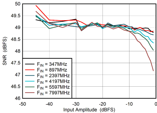
5-57. DES Mode: SNR vs Input Amplitude
