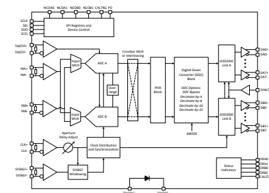
ADC12DJ4000RF ブロック図
