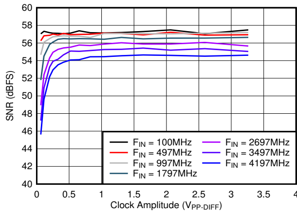
8-37. SNR vs A_{CLK}
