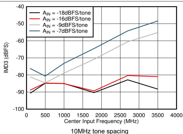
FIG 8-75. IMD3 vs F_{IN}
