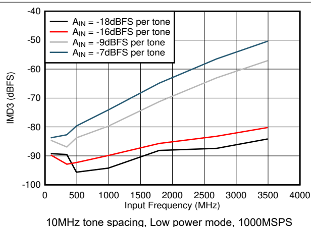
FIG 8-76. IMD3 vs F_{IN}
