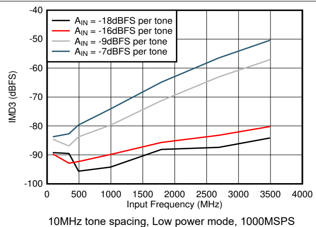
FIG 7-76. IMD3 vs F_{IN}
