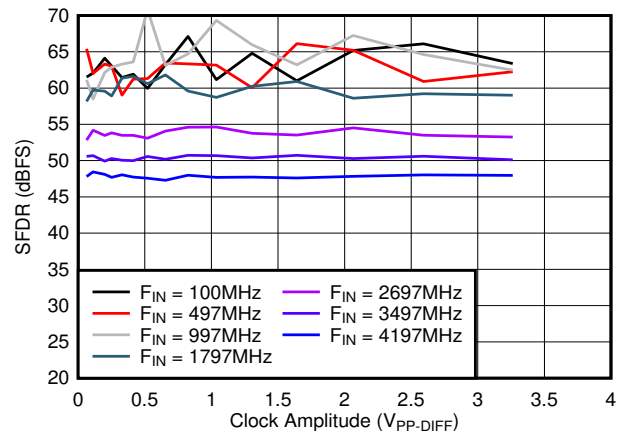
7-36. SFDR vs A_{CLK}
