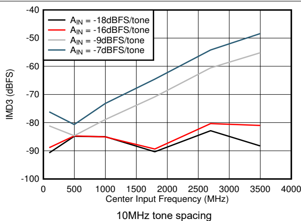
FIG 7-75. IMD3 vs F_{IN}
