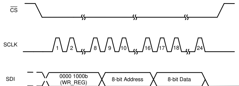
図 7-9. Register Write Operation
