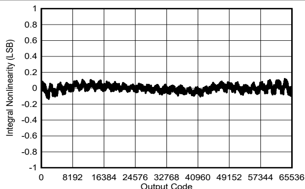
図 6-19. 標準 INL
