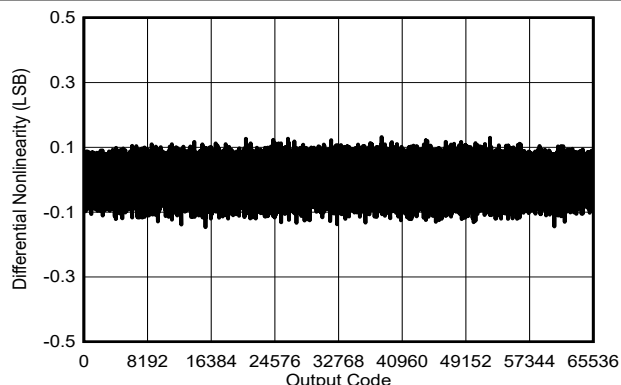
図 6-20. 標準 DNL : ADS9229
