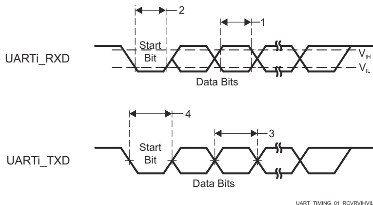
図 6-110. UART のタイミング要件およびスイッチング特性
