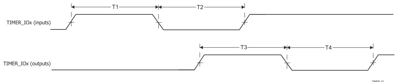
図 6-109. タイマのタイミング要件およびスイッチング特性
