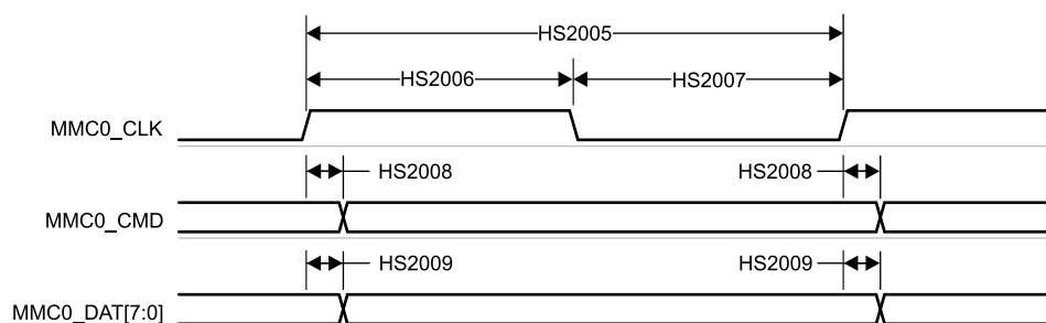
図 6-73. MMC0 – HS200 モード – 送信モード
