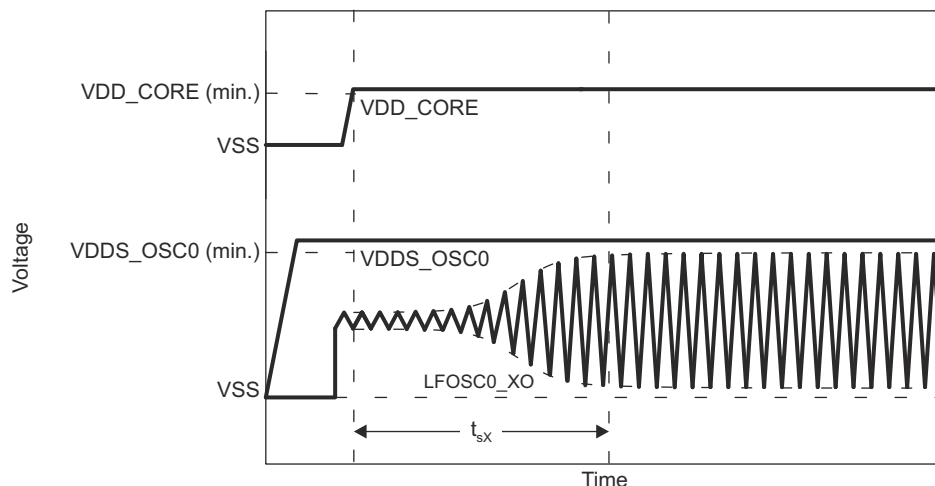
図 6-27. LFOSC0 スタートアップ時間
