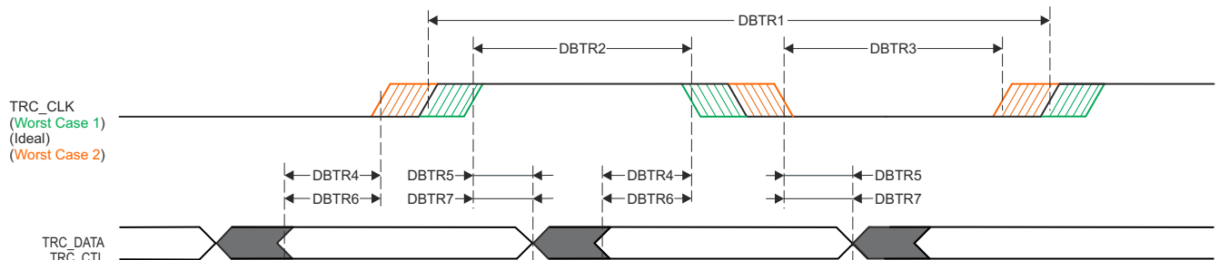
図 6-43. トレースのスイッチング特性
