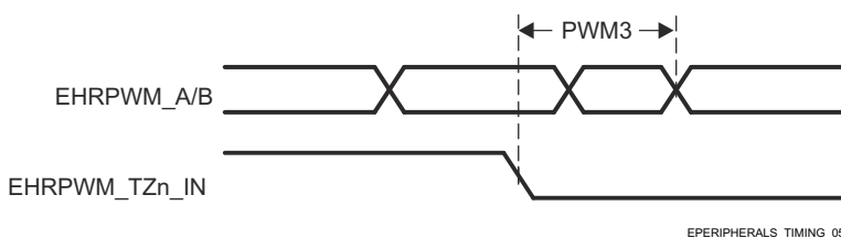
図 6-47. EHRPWM_TZn_IN から EHRPWM_A/B 強制へのスイッチング特性
