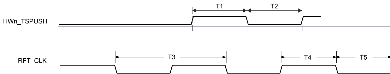
図 6-36. CPTS のタイミング要件
