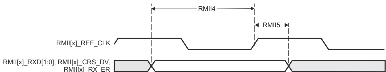
図 6-32. CPSW3G RMII[x]_RXD[1:0]、RMII[x]_CRS_DV、RMII[x]_RX_ER のタイミング要件 – RMII モード
