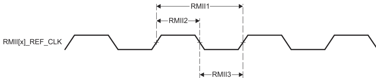
図 6-23. CPSW3G RMII[x]_REF_CLK のタイミング要件 - RMII モード
