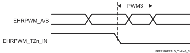
図 6-33. EHRPWM_TZn_IN から EHRPWM_A/B 強制へのスイッチング特性
