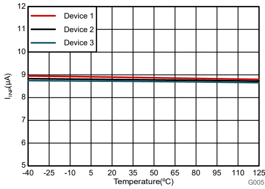
図 6-12. 入力電流と温度との関係
