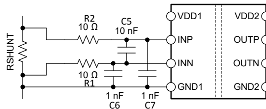
図 8-2. 差動入力フィルタ
