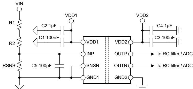
図 8-5. AMC0x30D のデカップリング
