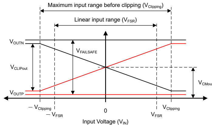
図 7-2. AMC0x30D の入力から出力への伝達曲線
