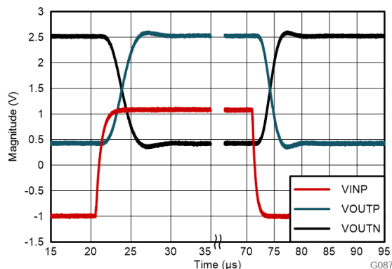
図 8-4. AMC0x30D のステップ応答
