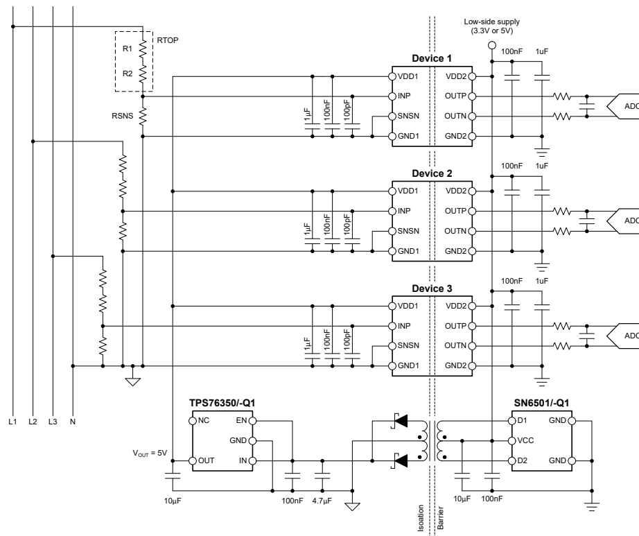
図 8-1. 代表的なアプリケーションで使用 AMC0x30D
