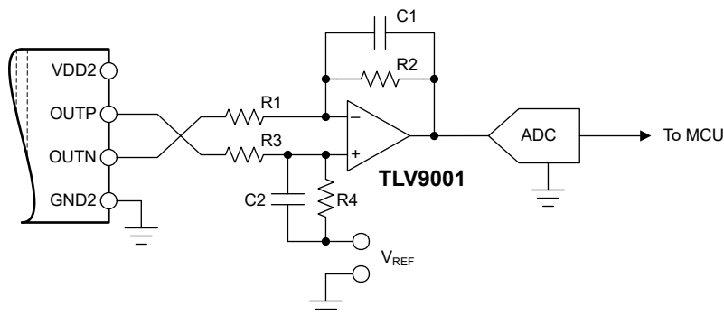
図 8-3. AMC0x30D 出力をシングルエンド入力 ADC に接続する
