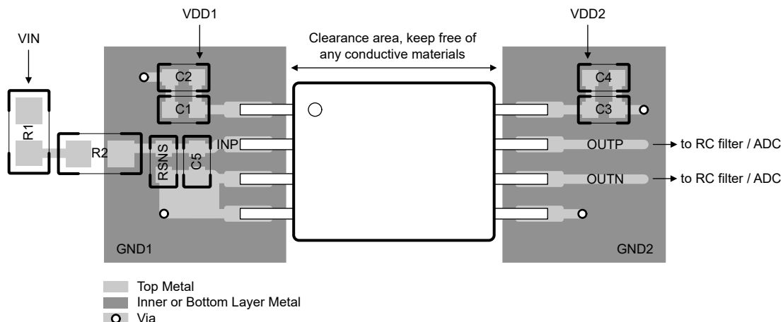
図 8-6. AMC0x30D の推奨レイアウト
