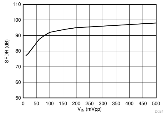
図 6-29. スプリアスフリー ダイナミック レンジと入力信号振幅との関係
