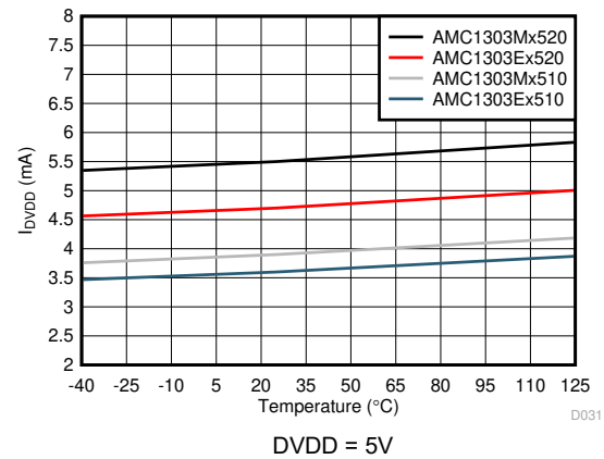
図 6-39. コントローラ側電源電流と温度との関係
