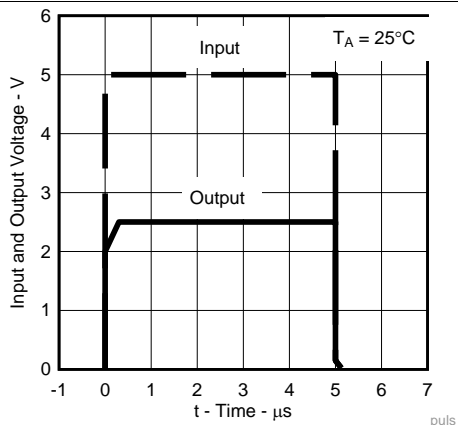
図 11. パルス応答
