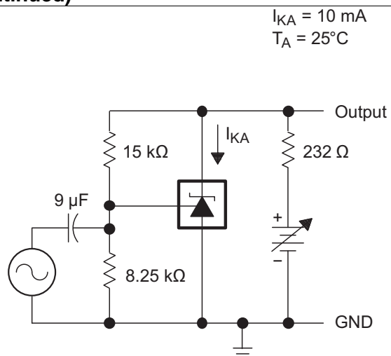
図 8. 電圧増幅のテスト回路
