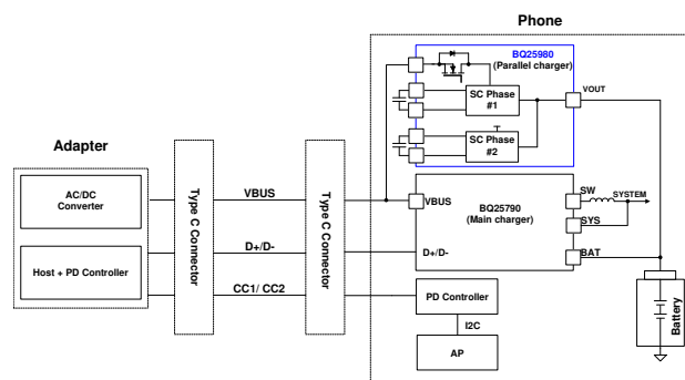
簡略回路図
