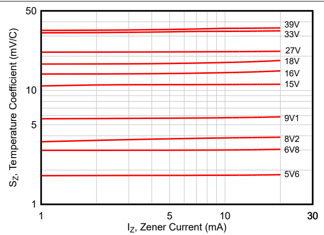
図 6-2. 温度係数
