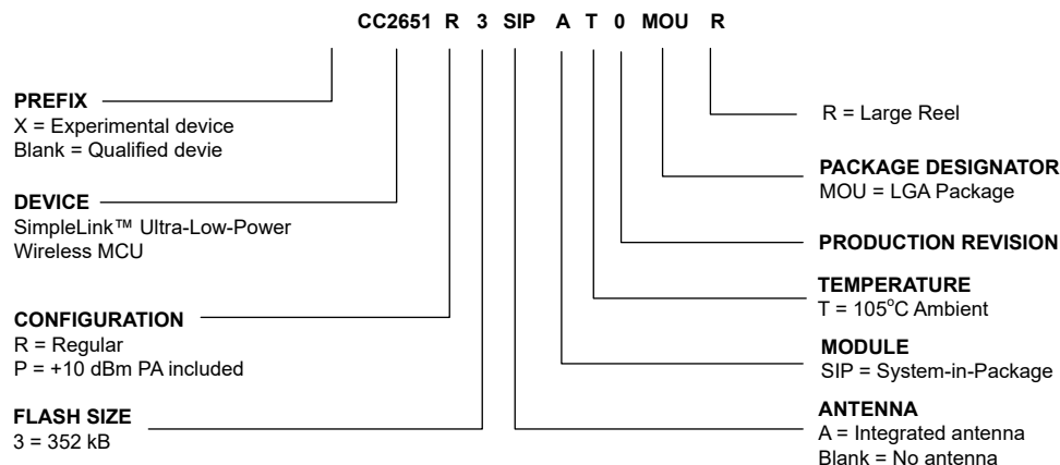
12-1. Device Nomenclature
