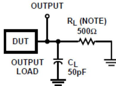
図 4-3. PROPAGATION DELAY TIMES
