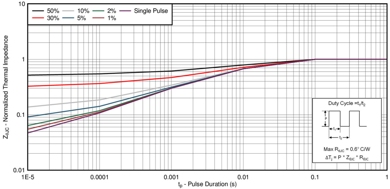
図 4-1. 過渡熱抵抗
