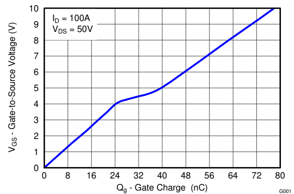
ゲート電荷
