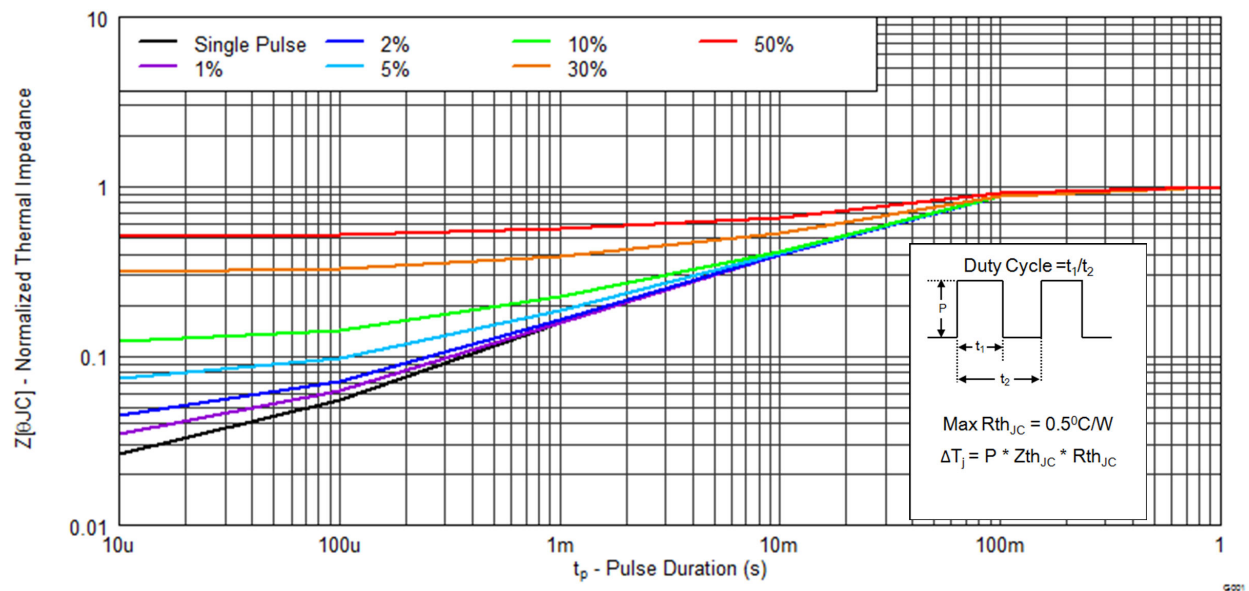
図 4-1. Transient Thermal Impedance
