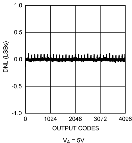
図 5-3. DNL vs Output Code
