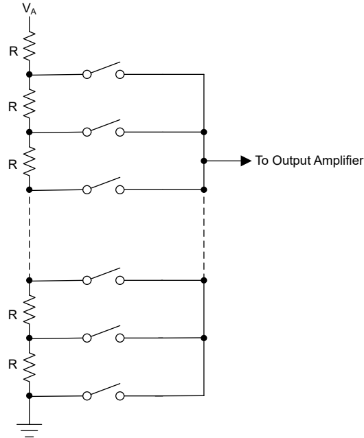
图 6-1. DAC Resistor String
