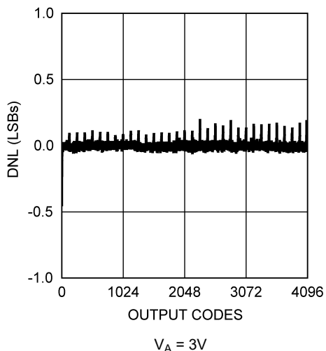
図 5-2. DNL vs Output Code
