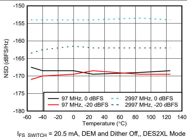
図 6-83. NSD vs Temperature
