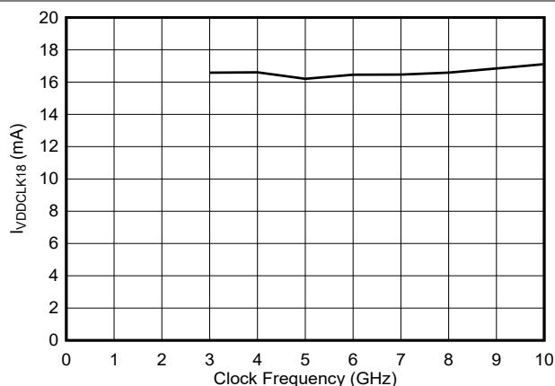
図 6-217. VDDCLK18 Current vs Clock Frequency
