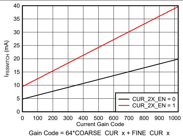
图 6-15. I_{\text{FS\_SWITCH}} vs Gain Code
