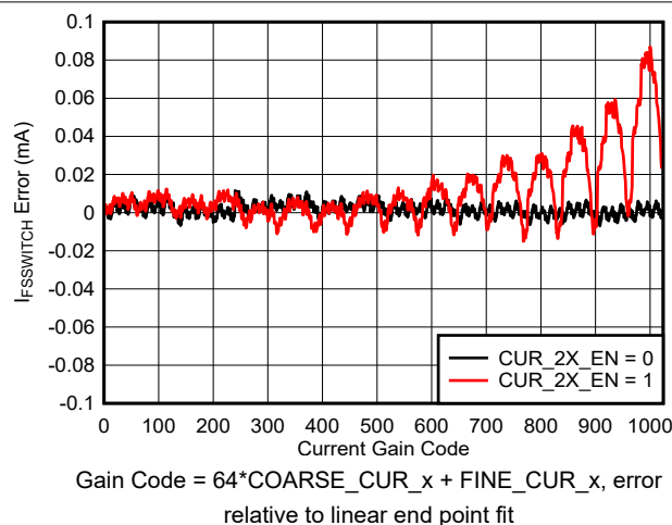
图 6-16. I_{\text{FS\_SWITCH}} Error vs Gain Code
