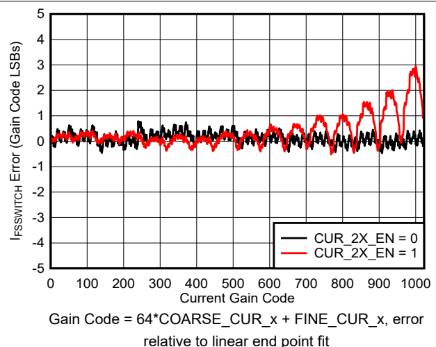
图 6-17. I_{\text{FS\_SWITCH}} Error vs Gain Code
