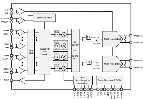
ブロック図
