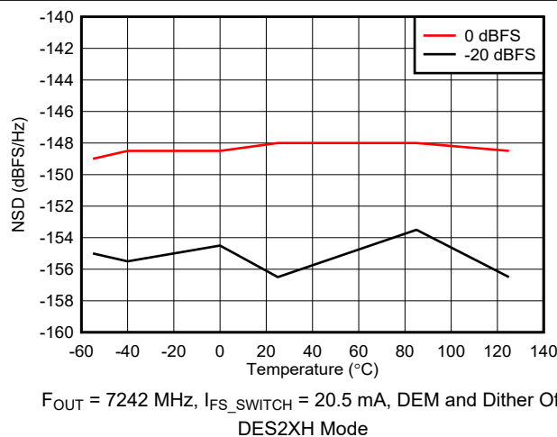
図 6-84. NSD vs Temperature
