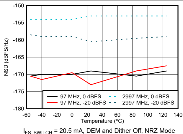
図 6-81. NSD vs Temperature
