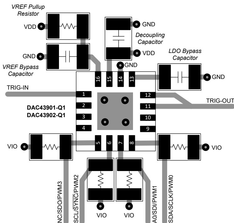
图 8-4. Layout Example
