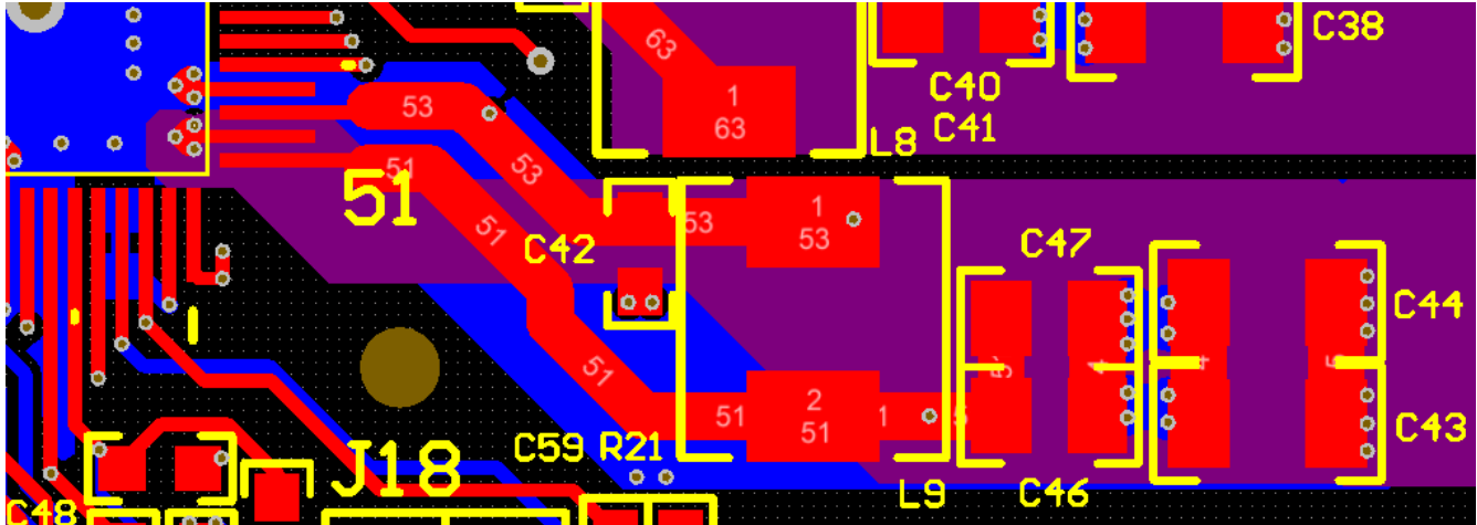
☒ 7-7. Practical Layout
