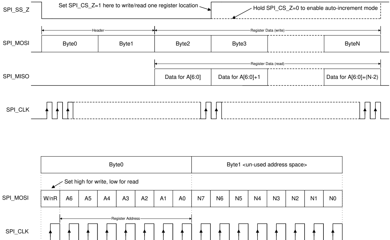
図 6-10. SPI Protocol
