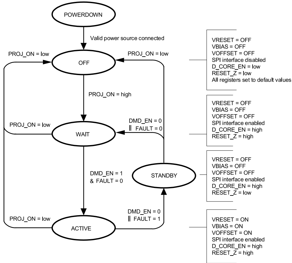
図 6-9. State Diagram
