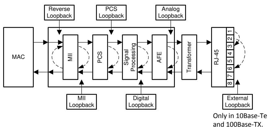
图 7-11. Loopbacks
