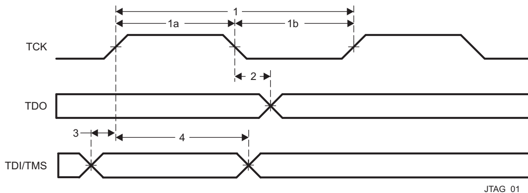
图 7-94. JTAG Timing
