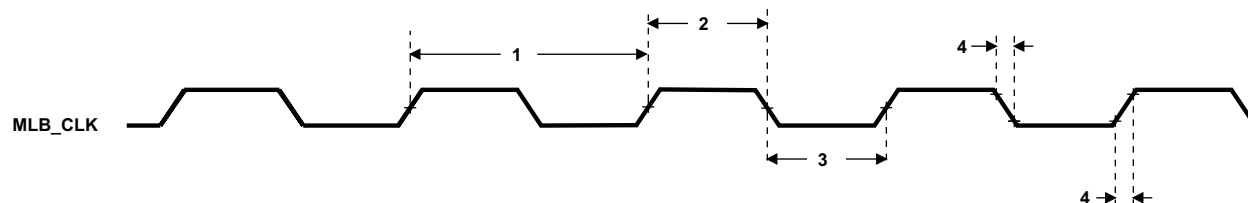
图 7-61. MLB_CLK Timing
