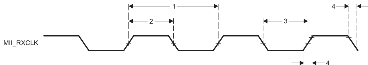
图 5-125. PRU-ICSS MII[x]_RXCLK Timing
