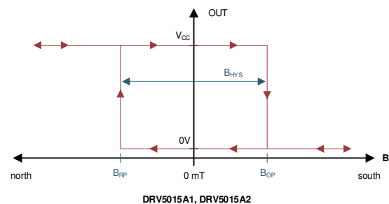
磁気応答
