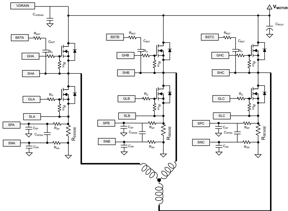
図 8-1. DRV8334-Q1 の代表的なアプリケーション図
