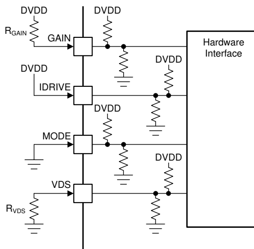
FIG 28. Hardware Interface
