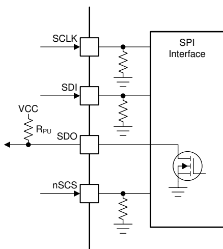
FIG 27. SPI
