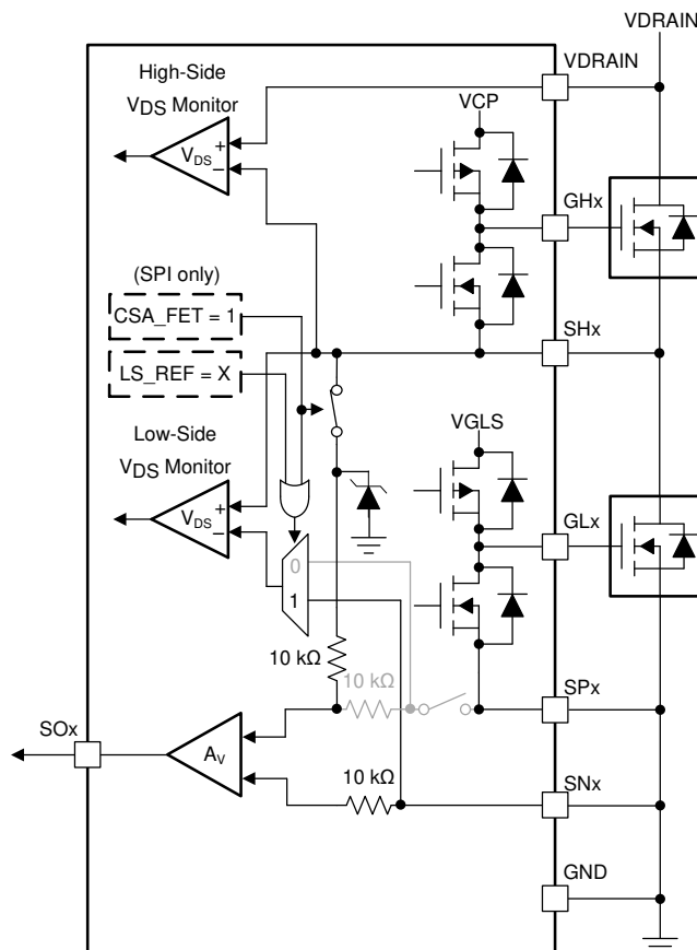
図 49. V_{DS} Sense Configuration
