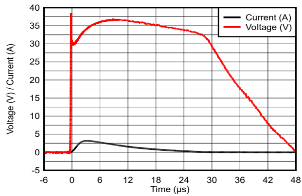
図 6-7. 8/20 \mu\text{s} のサージ応答
