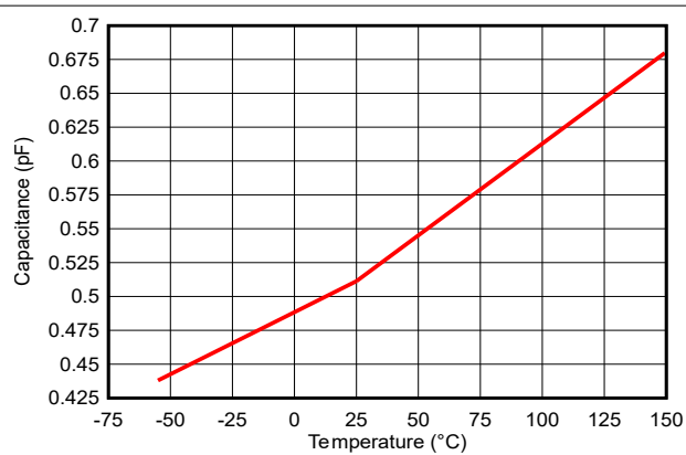
図 5-6. 静電容量と温度との関係
