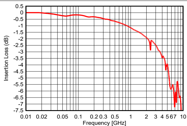
図 5-8. 挿入損失
