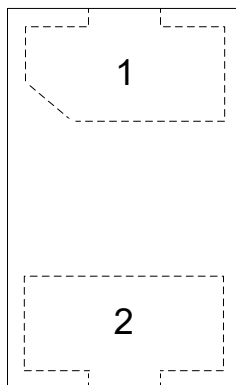
図 4-1. DPY パッケージ、2 ピン DFN1006 (上面図)
