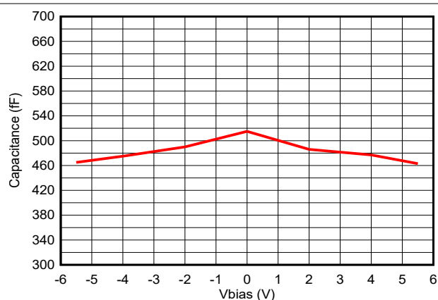
図 5-5. 静電容量とバイアス電圧との関係
