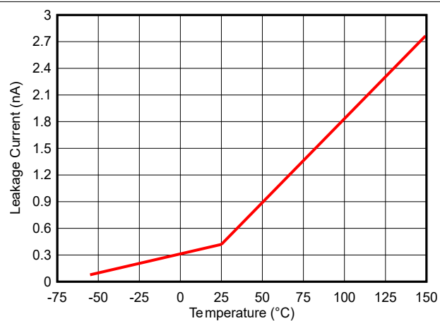
図 5-7. リーク電流と温度との関係
