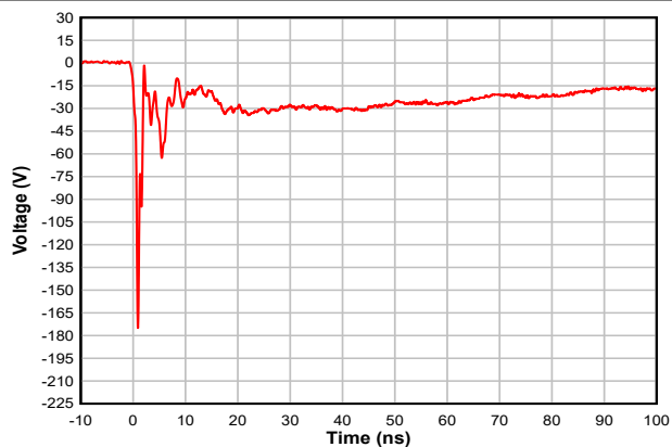
図 5-7. -8kV クランプ IEC 波形
