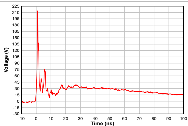
図 5-6. +8kV クランプ IEC 波形
