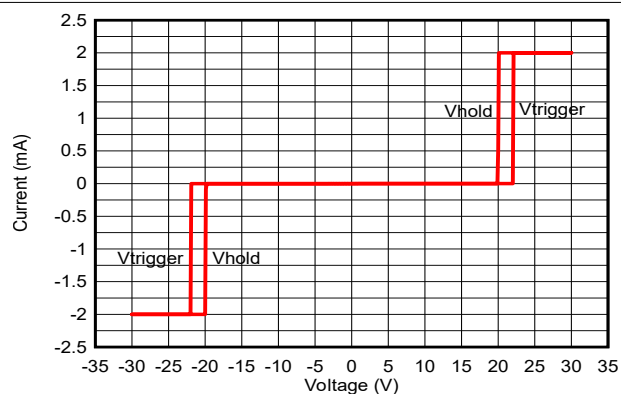
図 5-2. DC I-V 曲線
