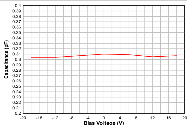
図 5-1. バイアス電圧と静電容量との関係
