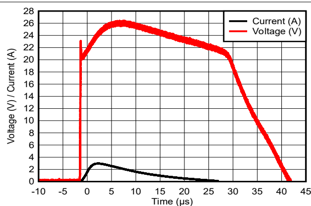
図 5-5. 8/20 \mu s サージ応答
