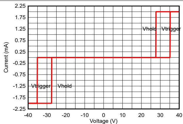
図 5-4. DC-IV Curve
