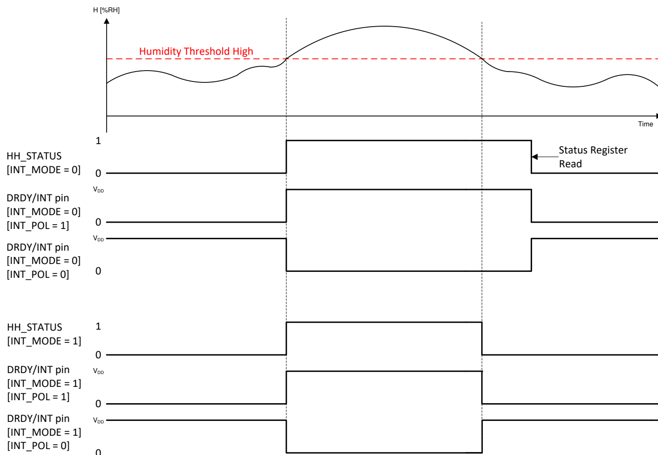
図 7-5. スレッシュホールド上の割り込み - 湿度 HIGH
