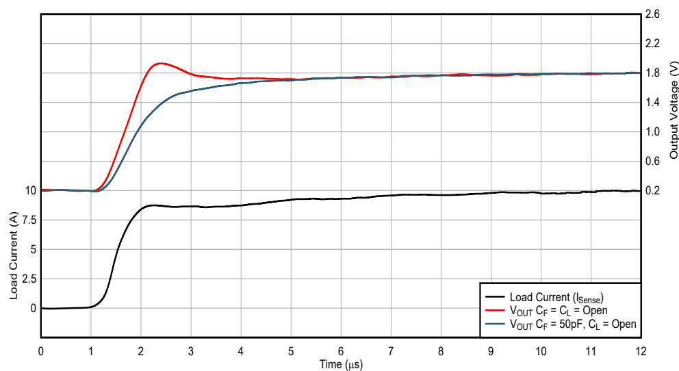
図 7-6. INA750x RISO デュアル フィードバックの前後での負荷ステップ応答により、可変ゲイン 1 を実現
