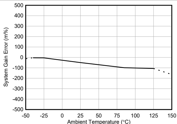
図 5-14. INA750B ゲイン誤差と温度との関係
