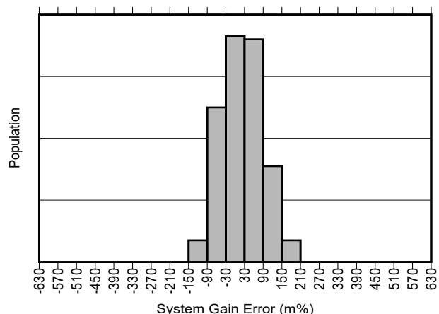
図 5-12. INA750B ゲイン誤差の製品分布
