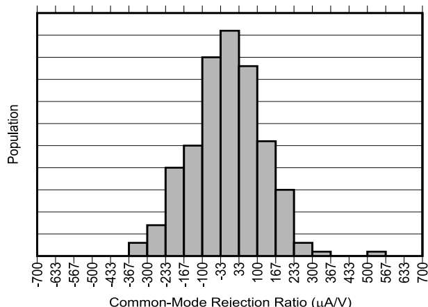
図 5-6. INA750B 同相除去比の製品分布
