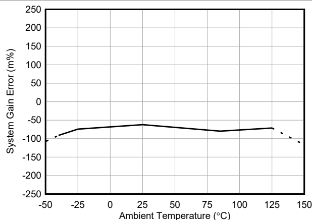
図 5-13. INA750A ゲイン誤差と温度との関係
