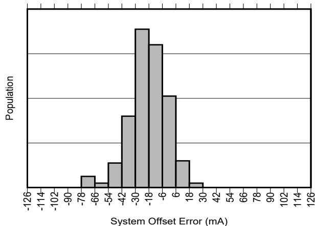
図 5-2. INA750B 入力オフセット電流の製品分布
