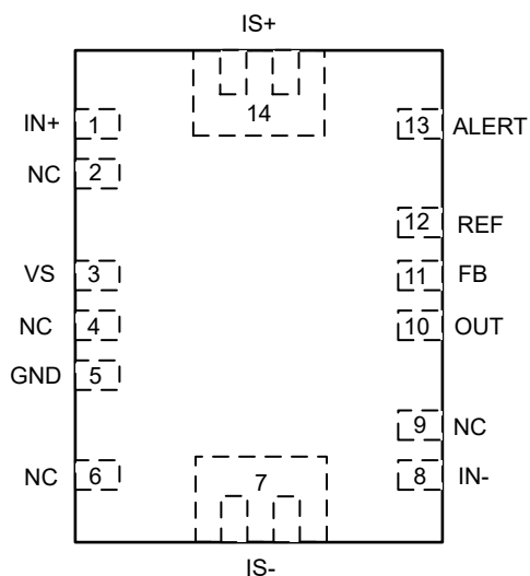
図 4-1. INA750x REM パッケージ VQFN 上面図
