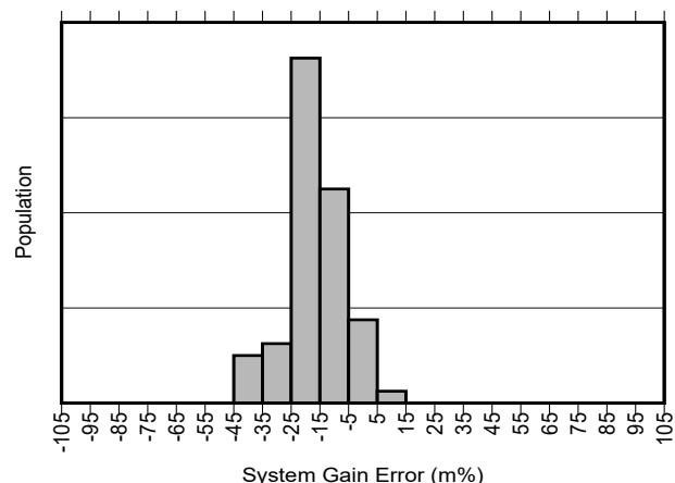
図 5-11. INA750A ゲイン誤差の製品分布
