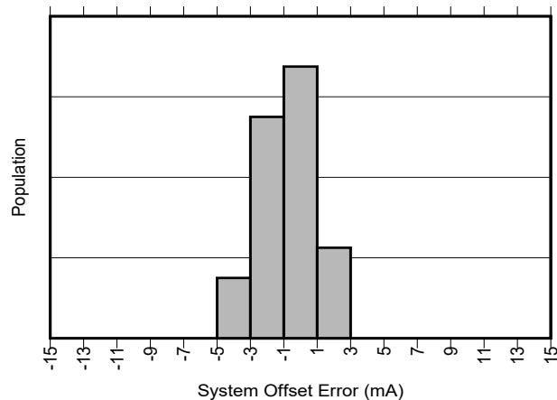
図 5-1. INA750A 入力オフセット電流の製品分布
