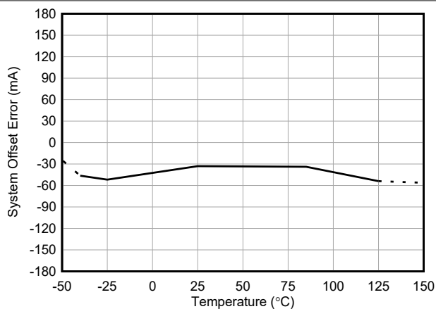
図 5-4. INA750B の入力オフセット電流と温度との関係
