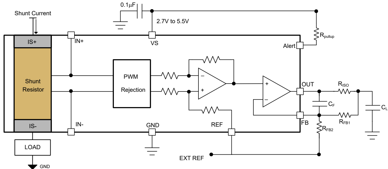
図 7-5. INA750x、RISO - デュアル フィードバック
