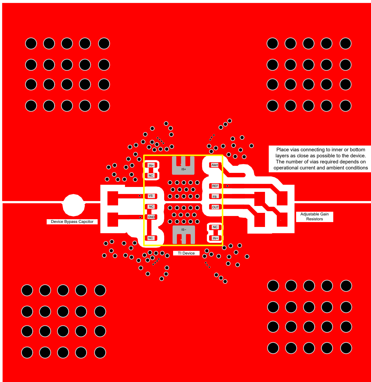
図 7-12. INA750x レイアウト例
