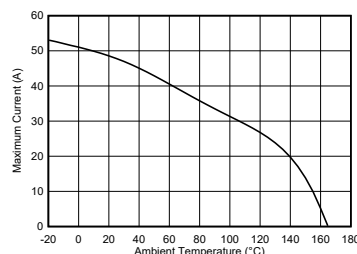
最大連続電流と周囲温度との関係
