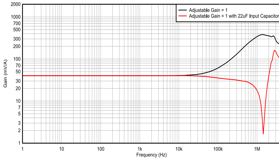
図 7-4. INA750x のゲインと、22 \mu F 入力コンデンサの追加前後の周波数との関係
