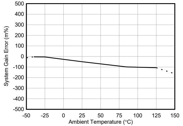
図 5-14. INA751B-Q1 ゲイン誤差と温度との関係
