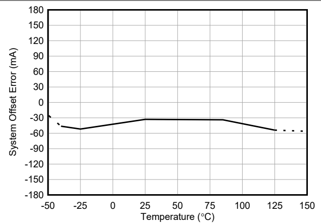
図 5-4. INA751B-Q1 の入力オフセット電流と温度との関係
