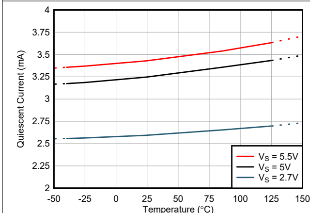
図 5-23. 静止電流と温度との関係
