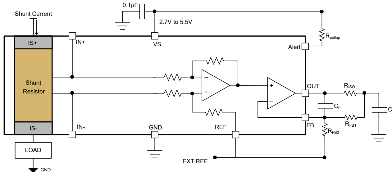
図 7-5. INA751x-Q1、RISO - デュアル フィードバック
