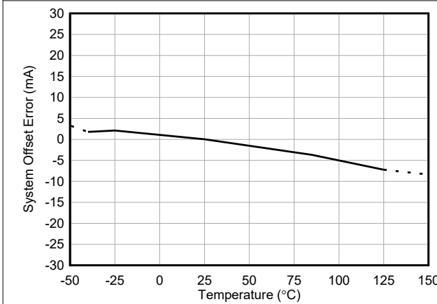
図 5-3. INA751A-Q1 の入力オフセット電流と温度との関係
