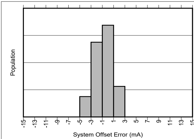
図 5-1. INA751A-Q1 入力オフセット電流の製品分布
