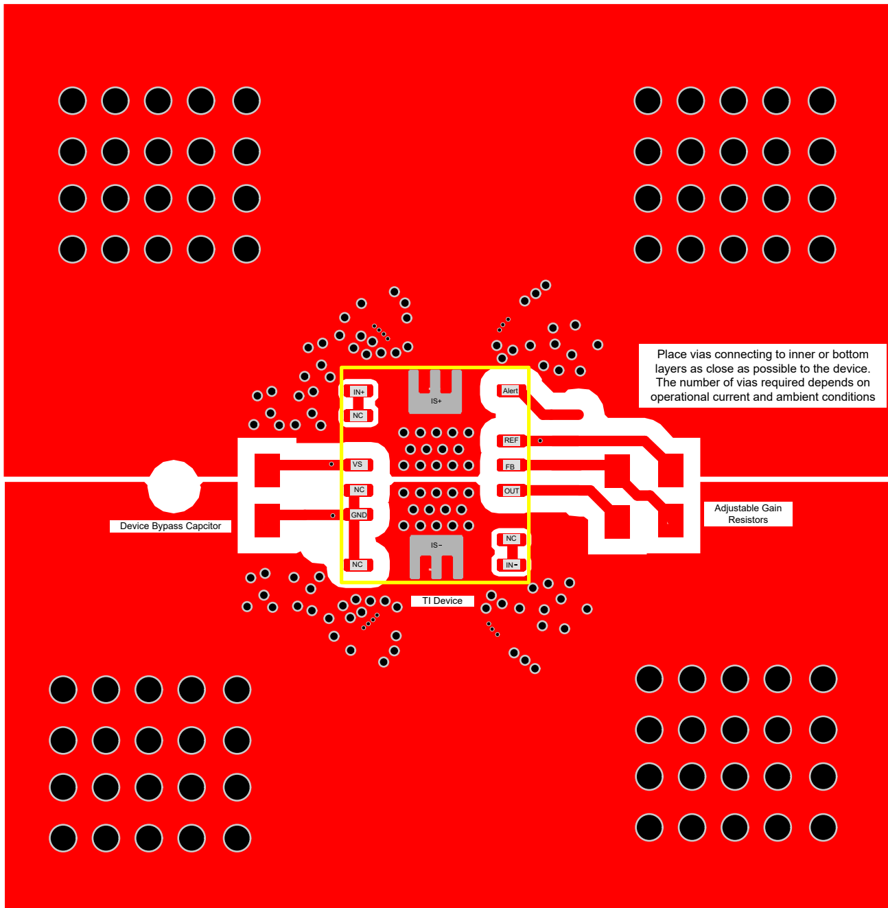
図 7-10. INA751x-Q1 レイアウト例
