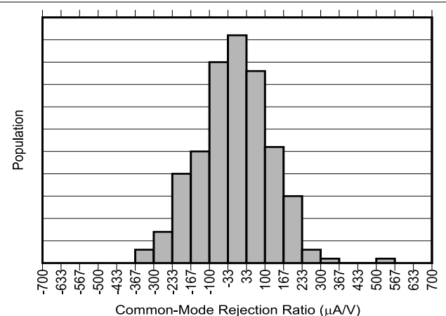
図 5-6. INA751B-Q1 同相除去比の製品分布
