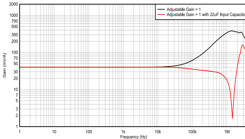
図 7-4. INA751x-Q1 のゲインと、22 \mu F 入力コンデンサの追加前後の周波数との関係
