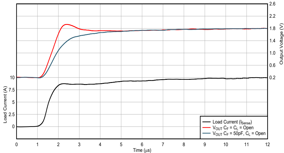
図 7-6. INA751x-Q1 RISO デュアル フィードバックの前後での負荷ステップ応答により、可変ゲイン 1 を実現
