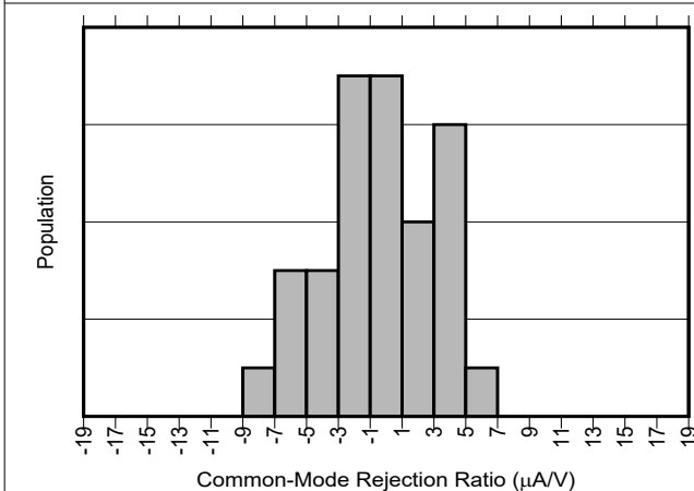
図 5-5. INA751A-Q1 同相除去比の製品分布
