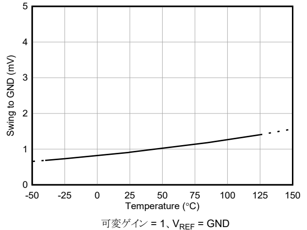
図 5-18. 出力電圧スイング Low と温度との関係
