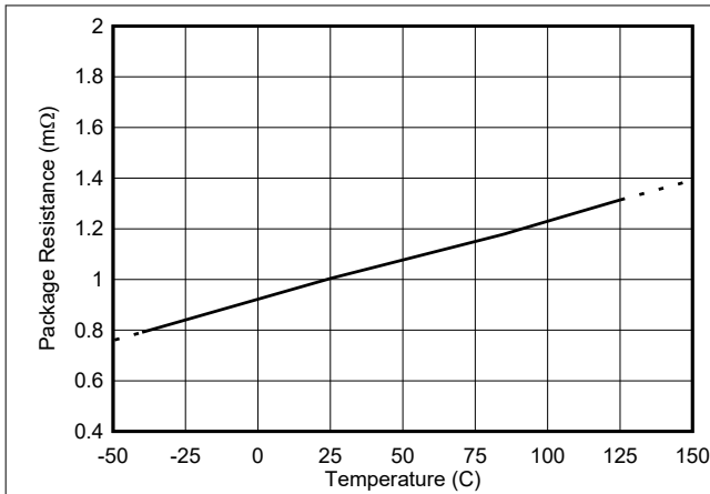
図 5-19. パッケージ抵抗と温度との関係
