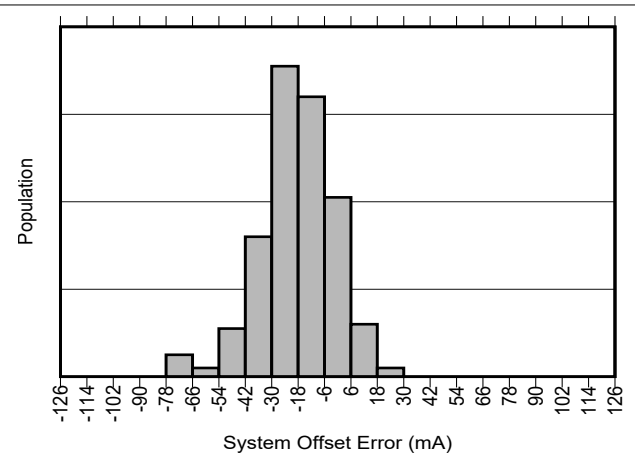
図 5-2. INA751B-Q1 入力オフセット電流の製品分布
