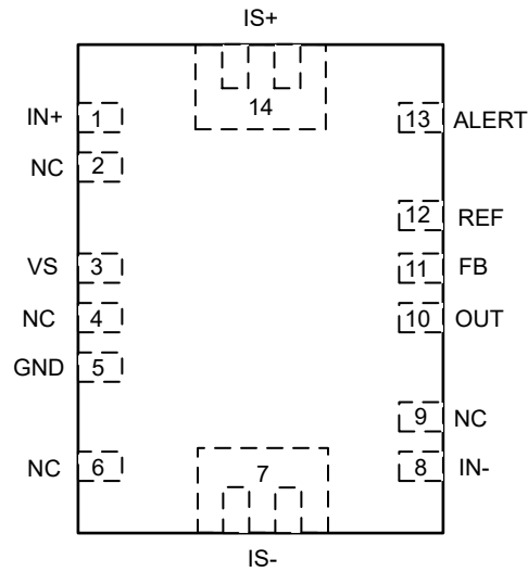
図 4-1. INA751x-Q1 REM パッケージ VQFN 上面図
