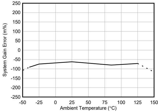
図 5-13. INA751A-Q1 ゲイン誤差と温度との関係
