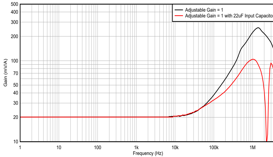
図 7-4. INA790x-Q1 のゲインと、22 \mu F 入力コンデンサの追加前後の周波数との関係
