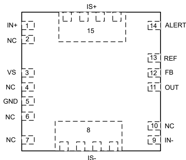
図 4-1. INA790x-Q1 ウェットブル DEK パッケージ 15 ピン VQFN 上面図
