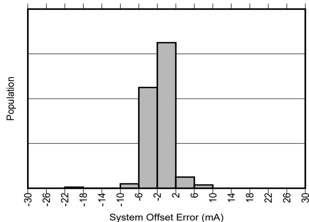
図 5-1. INA790A-Q1 入力オフセット電流の製品分布
