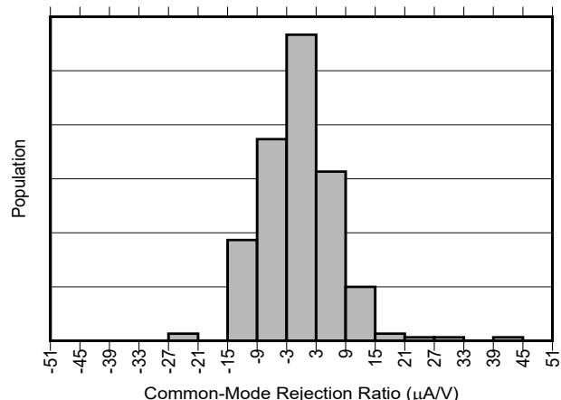
図 5-5. INA790A-Q1 同相除去比の製品分布
