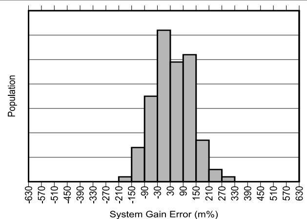
図 5-12. INA790B-Q1 ゲイン誤差の製品分布
