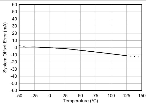
図 5-3. INA790A-Q1 の入力オフセット電流と温度との関係
