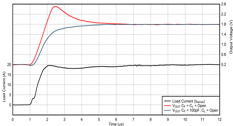
図 7-6. INA790x-Q1 RISO デュアル フィードバックの前後での負荷ステップ応答により、可変ゲイン 1 を実現
