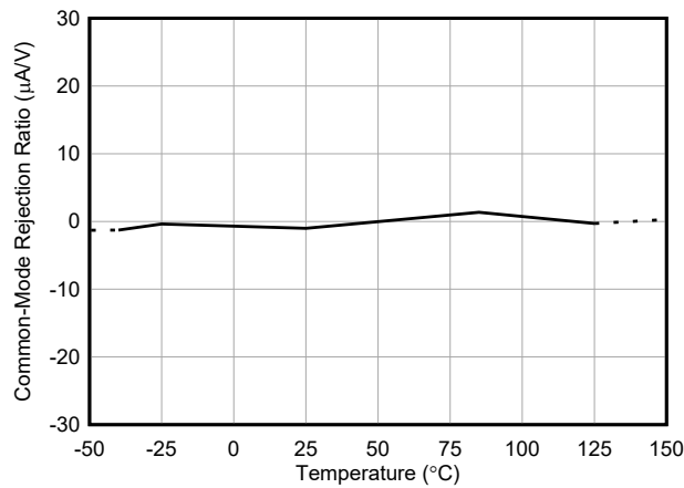
図 5-7. 同相除去比と温度との関係
