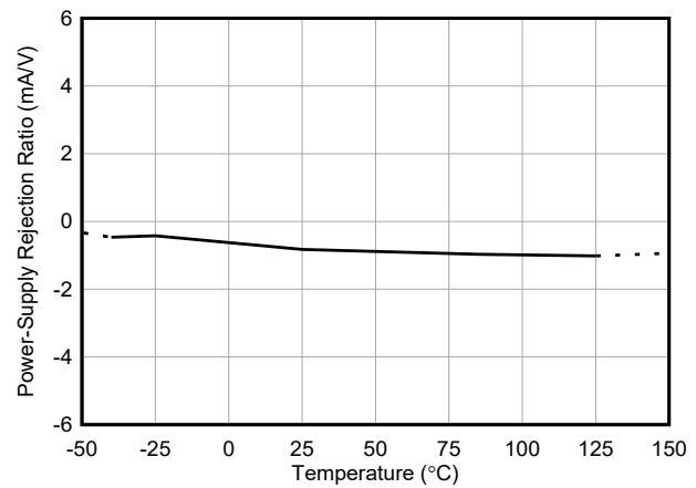
図 5-8. 電源除去比と温度との関係
