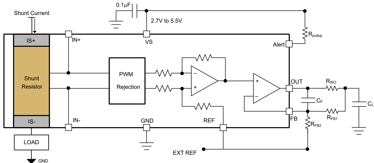
図 7-5. INA790x-Q1 、RISO - デュアル フィードバック
