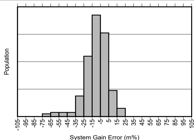
図 5-11. INA790A-Q1 ゲイン誤差の製品分布
