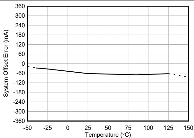
図 5-4. INA790B-Q1 の入力オフセット電流と温度との関係
