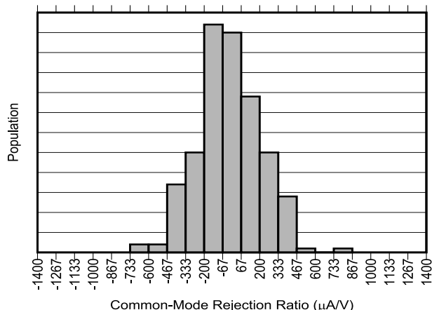
図 5-6. INA790B-Q1 同相除去比の製品分布
