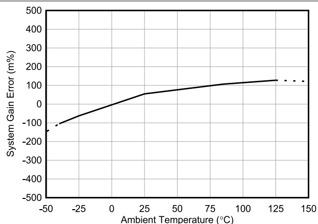
図 5-14. INA790B-Q1 ゲイン誤差と温度との関係
