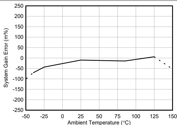
図 5-13. INA790A-Q1 ゲイン誤差と温度との関係
