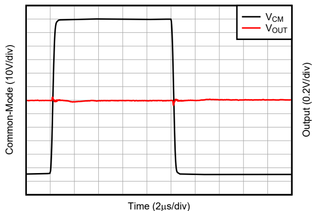
図 5-34. -4V ~ 110V 同相モード ステップ過渡応答
