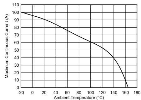
最大連続電流と周囲温度との関係
