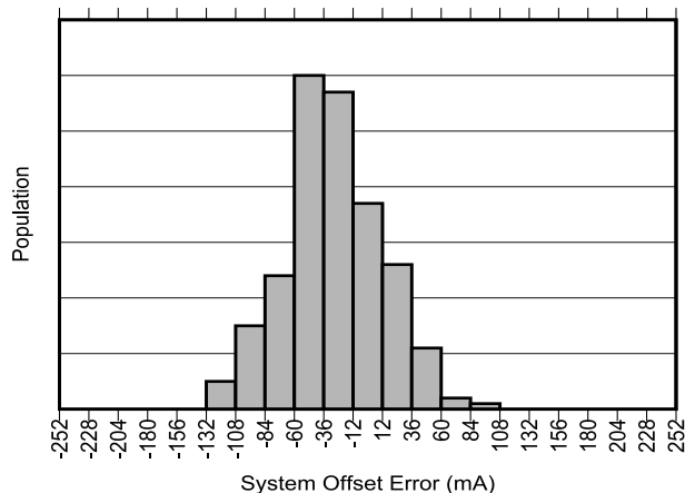
図 5-2. INA790B-Q1 入力オフセット電流の製品分布
