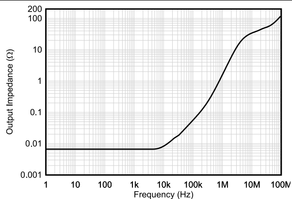
図 7-32. 開ループ出力インピーダンスと周波数との関係
