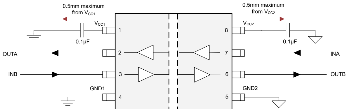
図 9-2. ISO602x の一般的な回路例
