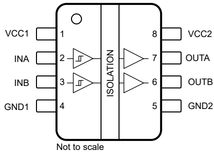
図 5-1. ISO6020H および ISO6020L の上面図
