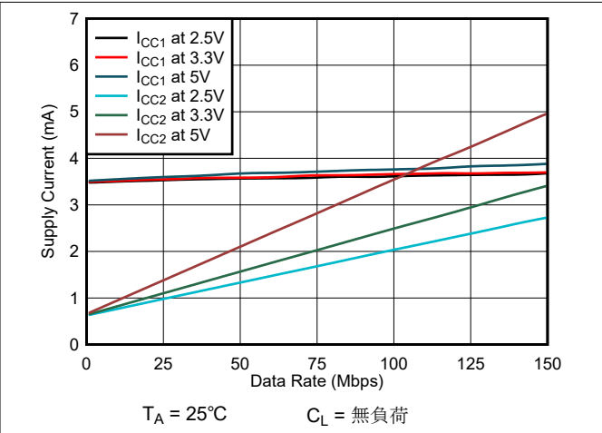
図 6-6. ISO6420-Q1 または ISO6420F-Q1 の消費電流とデータレートとの関係 (無負荷時)
