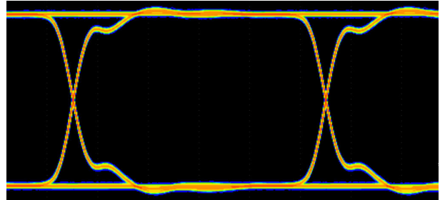
図 9-4. ISO642x-Q1 アイダイアグラム (100Mbps PRBS 2 16 - 1、3.3V、25°C)
