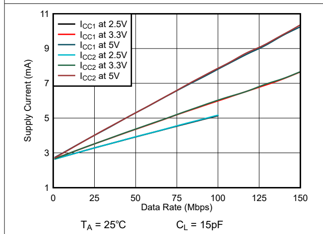
図 6-7. ISO6421-Q1 または ISO6421F-Q1 の消費電流とデータレートとの関係 (15pF 負荷時)
