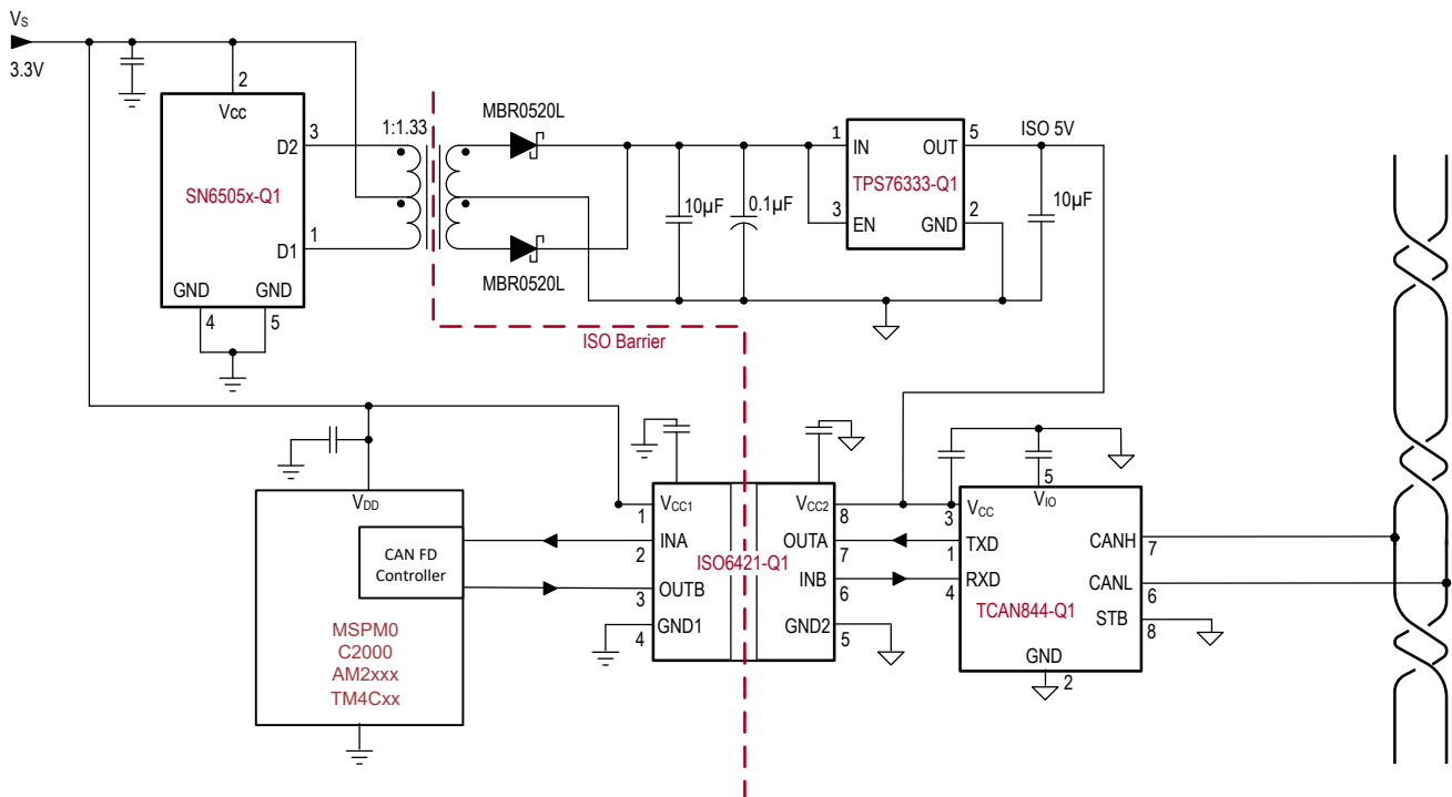
図 9-1. 2 チャンネルの代表的なアプリケーション
