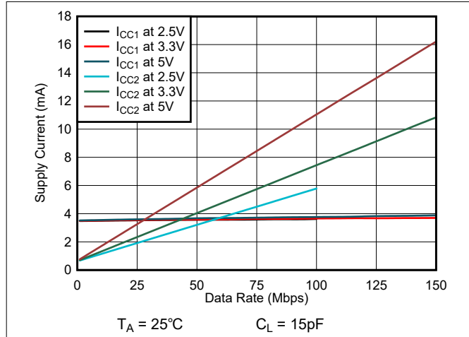
図 6-5. ISO6420-Q1 または ISO6420F-Q1 の消費電流とデータレートとの関係 (15pF 負荷時)
