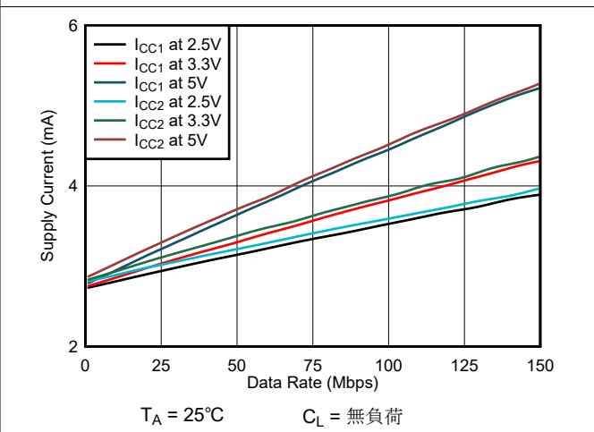
図 6-8. ISO6421-Q1 または ISO6421F-Q1 の消費電流とデータレートとの関係 (無負荷時)
