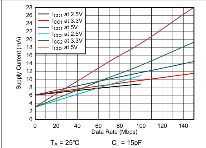
図 6-9. ISO6441 または ISO6441F の消費電流とデータレートとの関係 (15pF 負荷時)
