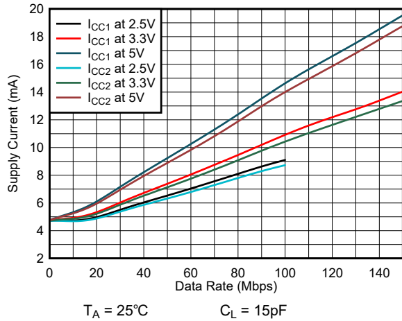
図 6-11. ISO6442 または ISO6442F の消費電流とデータレートとの関係 (15pF 負荷時)
