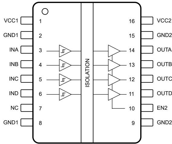
図 5-1. ISO6440 および ISO6440F の上面図
