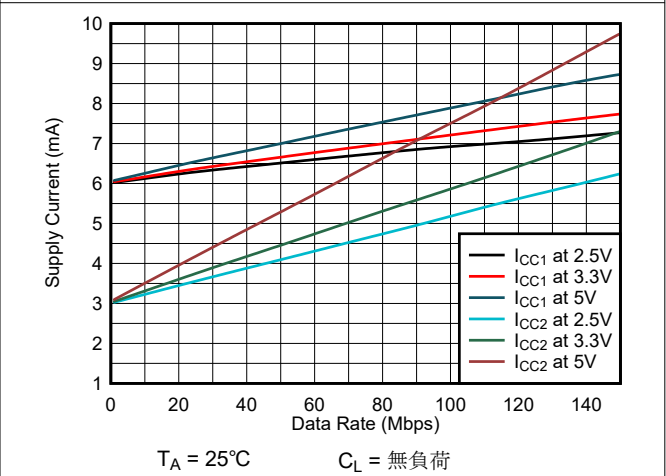
図 6-10. ISO6441 または ISO6441F の消費電流とデータレートとの関係 (無負荷時)
