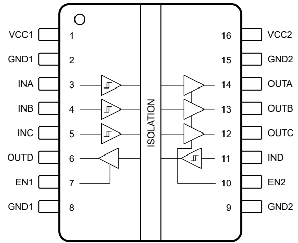
図 5-2. ISO6441 および ISO6441F の上面図
