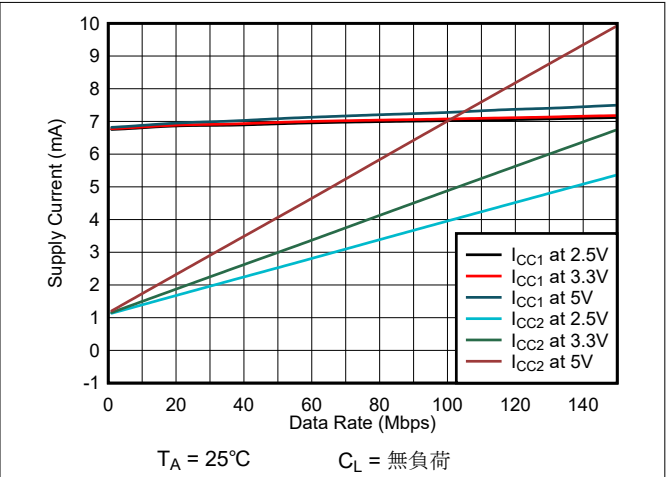
図 6-8. ISO6440 または ISO6440F の消費電流とデータレートとの関係 (無負荷時)
