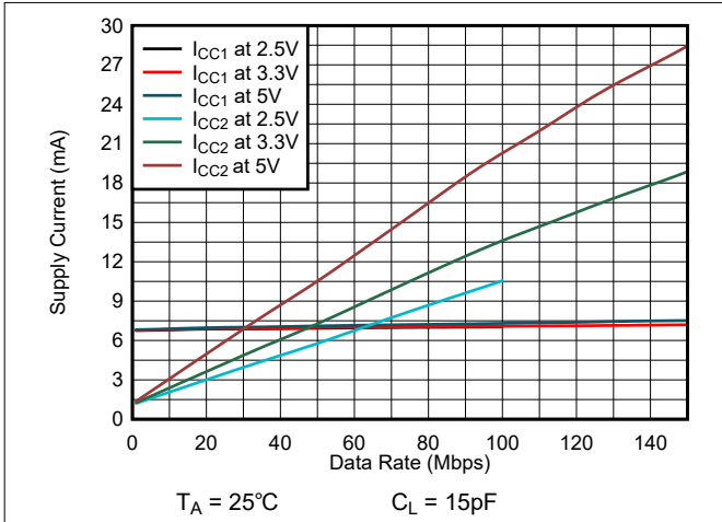
図 6-7. ISO6440 または ISO6440F の消費電流とデータレートとの関係 (15pF 負荷時)
