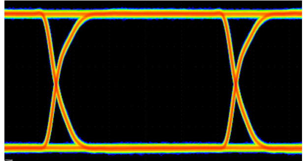
図 9-4. ISO646x アイダイアグラム (100Mbps PRBS 2^{16} - 1 、3.3V、25°C)
