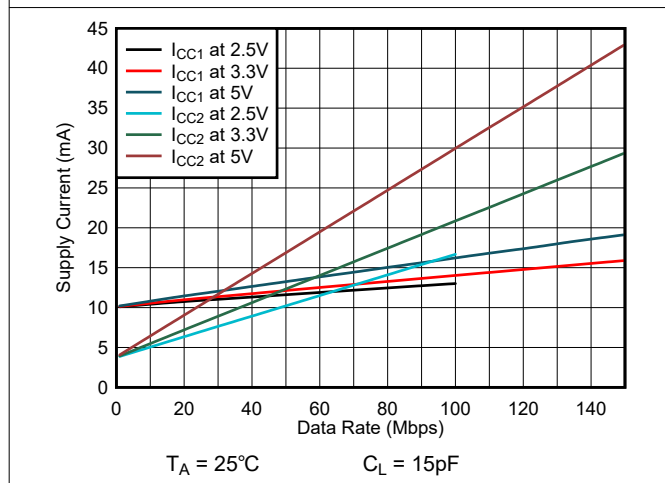
図 6-5. ISO6461 または ISO6461F の消費電流とデータレートとの関係 (15pF 負荷時)
