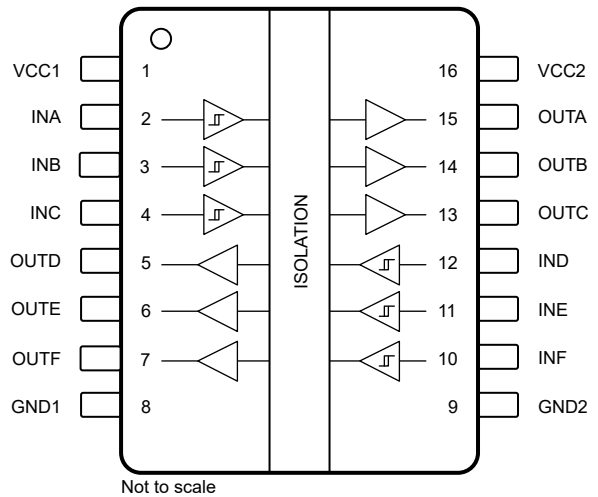
図 5-4. ISO6463 および ISO6463F の上面図
