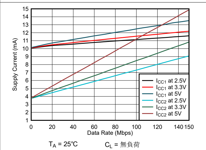
図 6-6. ISO6461 または ISO6461F の消費電流とデータレートとの関係 (無負荷時)
