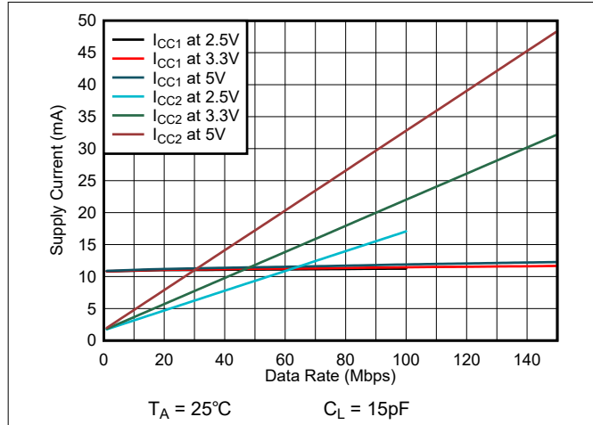
図 6-3. ISO6460 または ISO6460F の消費電流とデータレートとの関係 (15pF 負荷時)
