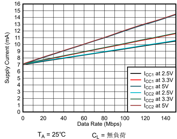
図 6-10. ISO6463 または ISO6463F の消費電流とデータレートとの関係 (無負荷時)
