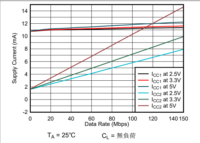
図 6-4. ISO6460 または ISO6460F の消費電流とデータレートとの関係 (無負荷時)
