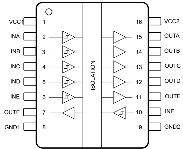
図 5-2. ISO6461 および ISO6461F の上面図
