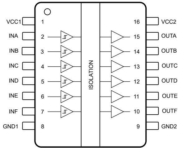
図 5-1. ISO6460 および ISO6460F の上面図
